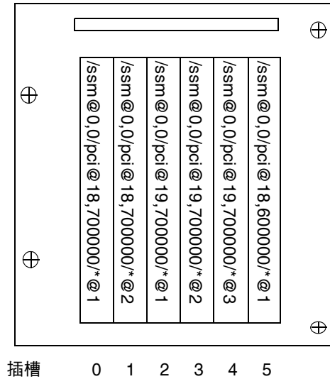
圖 10-1 IB6 的 Sun Fire 入門級中階系統 IB_SSC PCI 實體插槽指派
