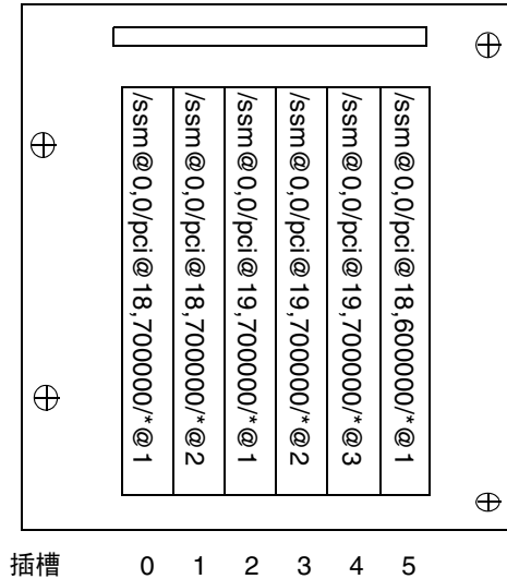
图 10-1 Sun Fire 入门级中型系统 IB_SSC PCI 物理插槽分配 (IB6)
