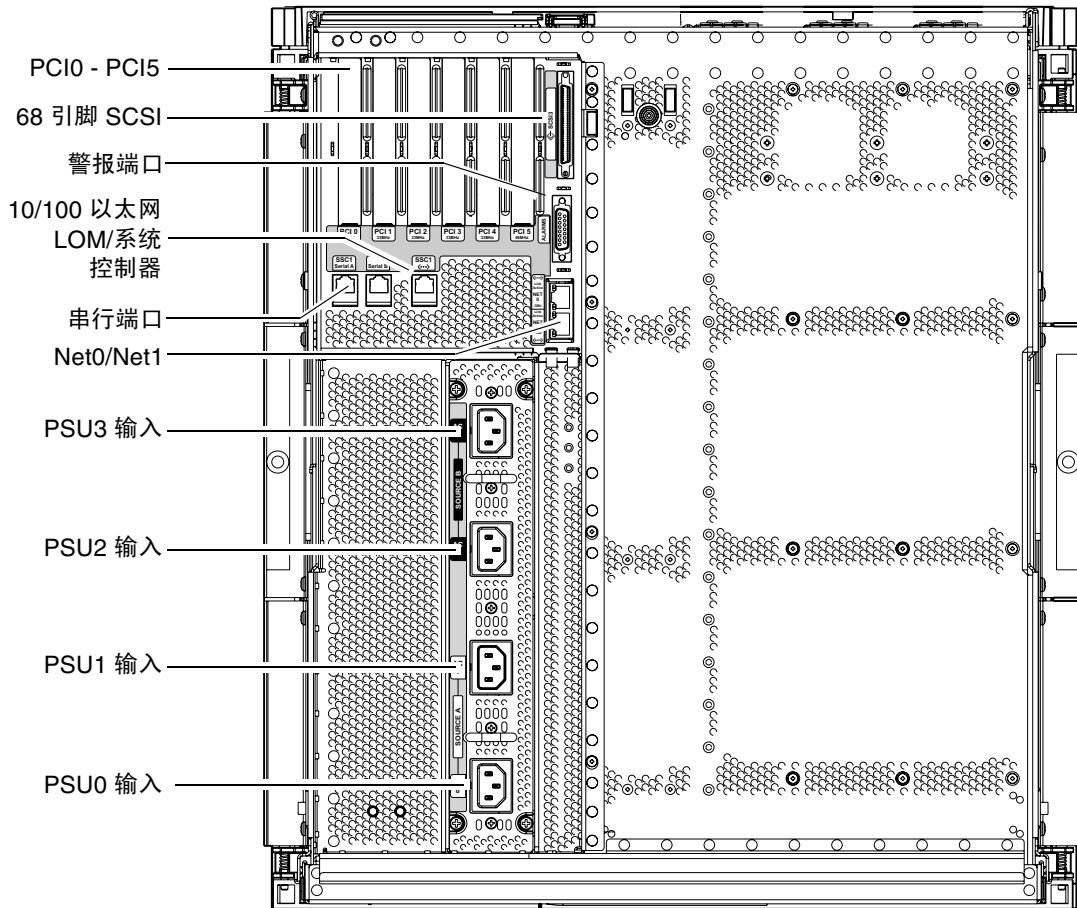
图 1-1 I/O 端口
