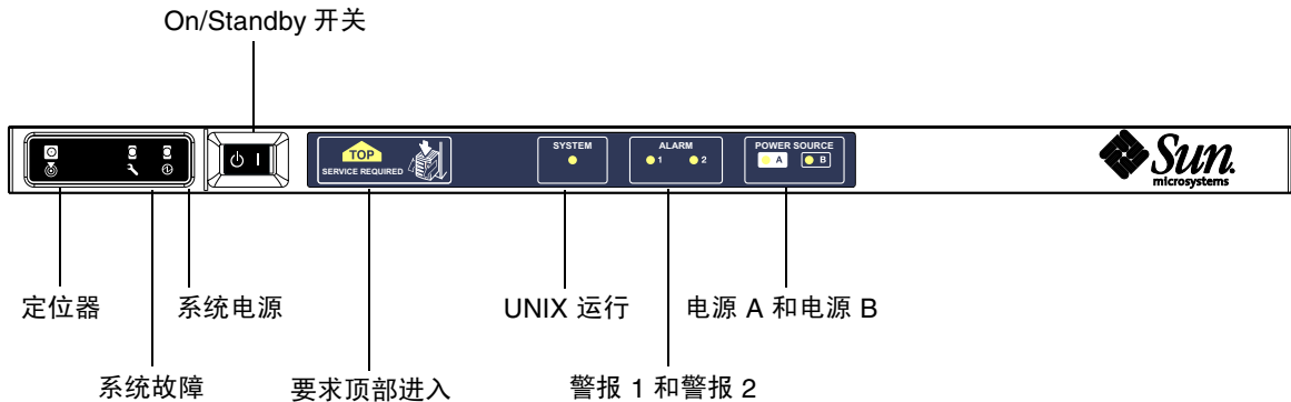
图 10-2 系统指示灯
