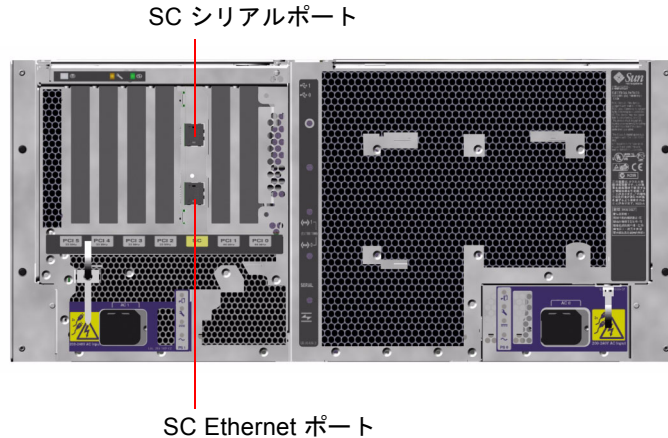
図 3-4 SC カードのポート
