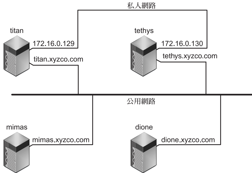
圖 5-1 網路介面
