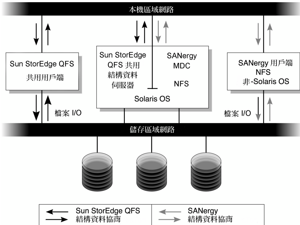
圖 9-1 使用 Sun StorEdge QFS 軟體和 SANergy 軟體的 SAN-QFS 檔案系統。
