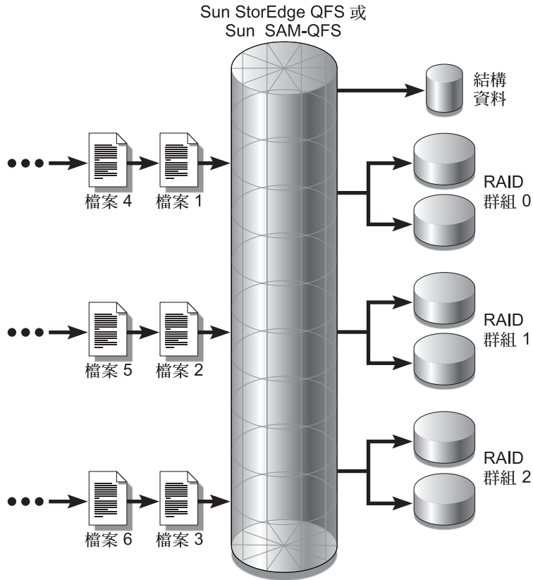
圖 2-5 Sun StorEdge QFS 循環資料分置群組
