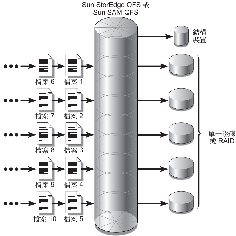
圖 2-2 使用 5 個裝置的循環 Sun StorEdge QFS 檔案系統
