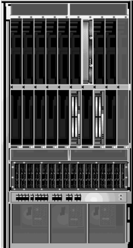
그림 5-6 Sun Fire 최고급 시스템 플랫폼 물리적 보기 — 전면
