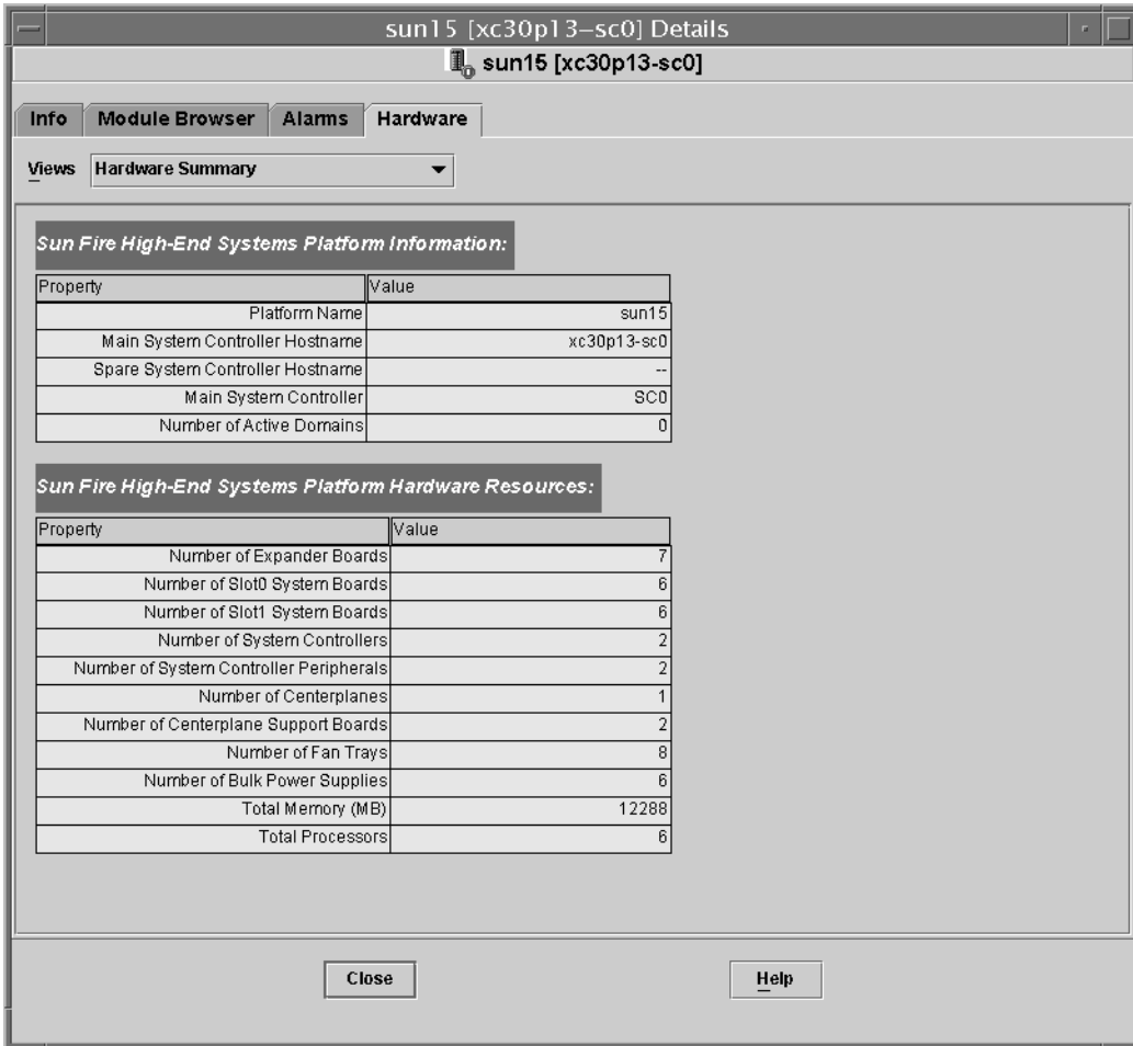
그림 5-1 Sun Fire 최고급 시스템 플랫폼에 대한 하드웨어 요약
