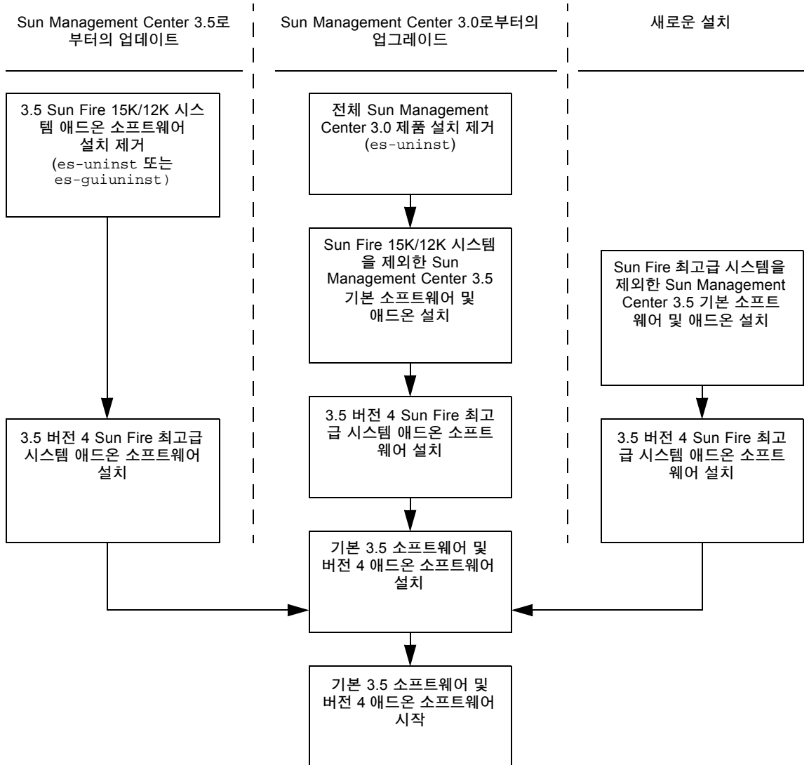
그림 2-1 설치 프로세스 흐름
