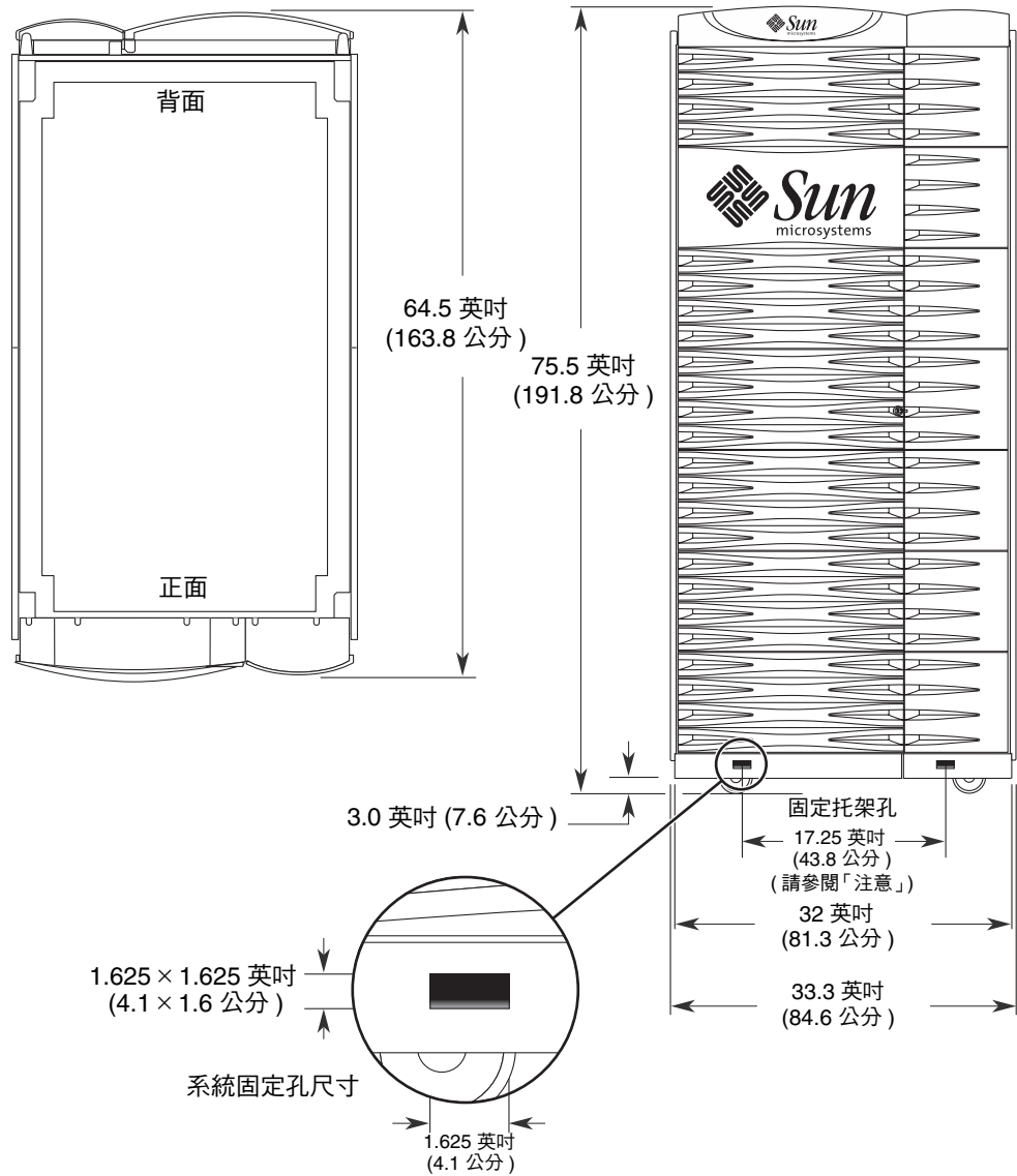
圖 1-4 Sun Fire E25K/E20K 系統機櫃尺寸
