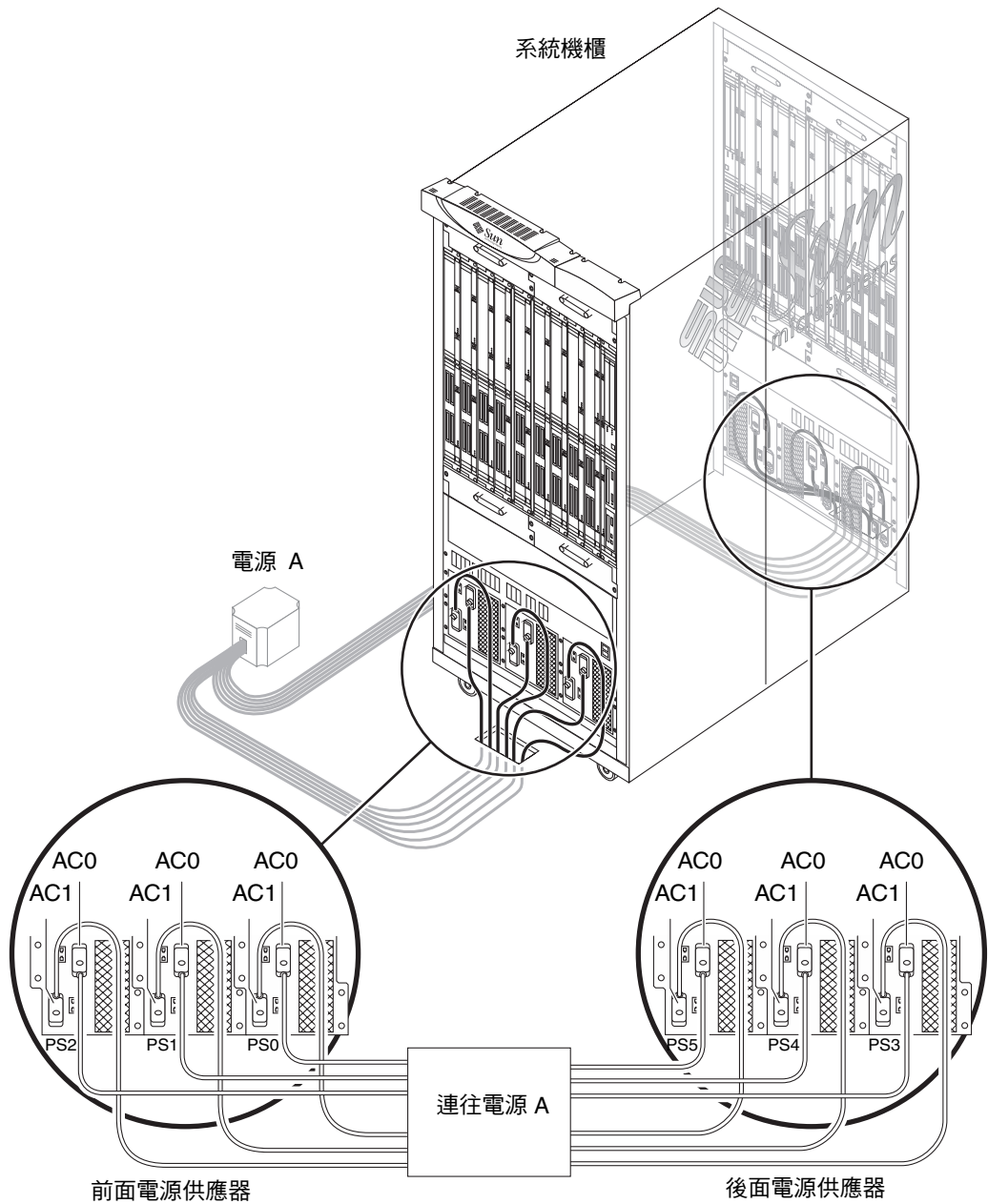
圖 3-2 Sun Fire E25K/E20K 系統電源連線 — 高可靠性電源、單一電源 (單電源)
