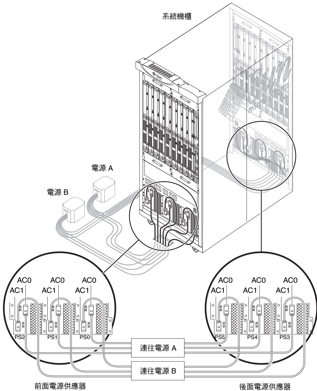
圖 3-1 Sun Fire E25K/E20K 系統電源連線 — 備援電源、雙電源 ( 電源 A 與 B )
