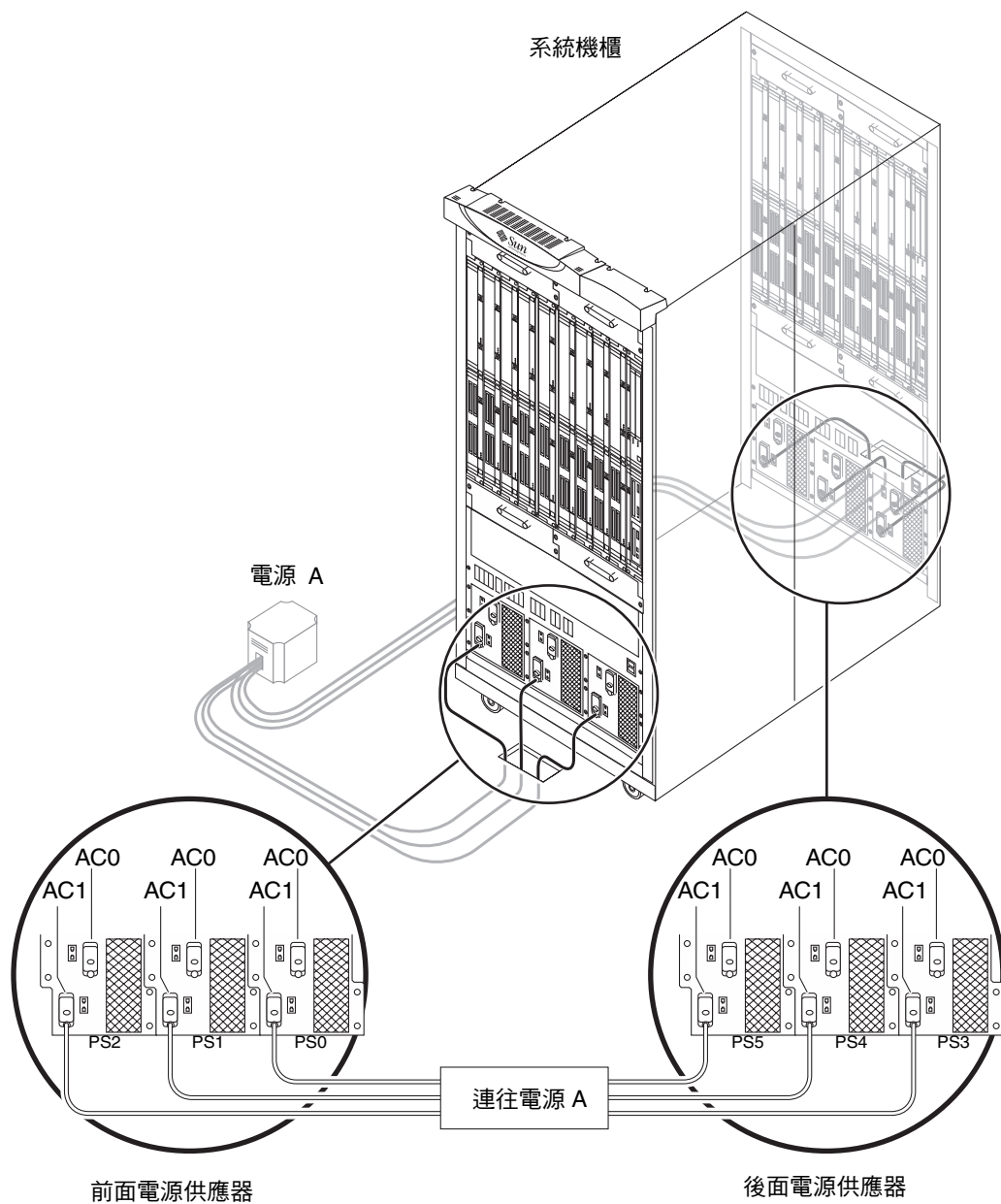
圖 3-3 Sun Fire E25K/E20K 系統電源連線 — 基本單一電源 (單電源、無備援、不建議使用)
