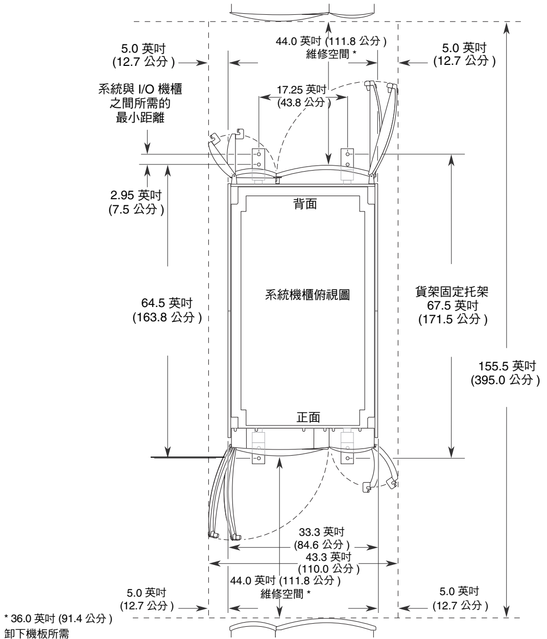
圖 1-5 Sun Fire E25K/E20K 系統機櫃淨空大小
