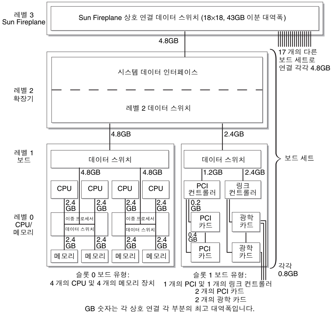
그림 4-4 데이터 상호 연결 레벨
