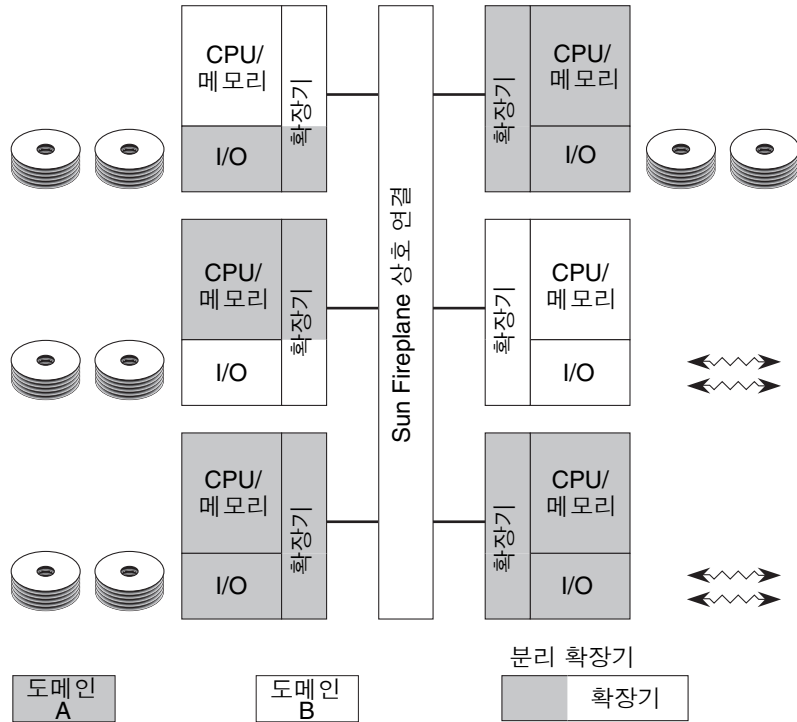
Sun Fire E25K 시스템을 나타낸 다이어그램
