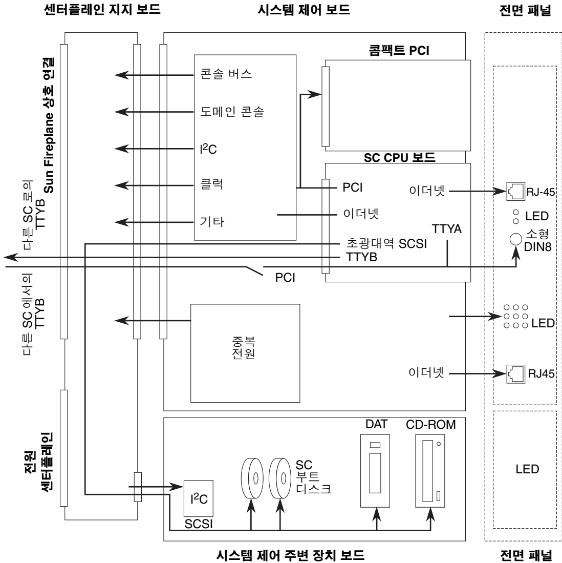
그림 5-6 시스템 컨트롤러 보드 레이아웃
