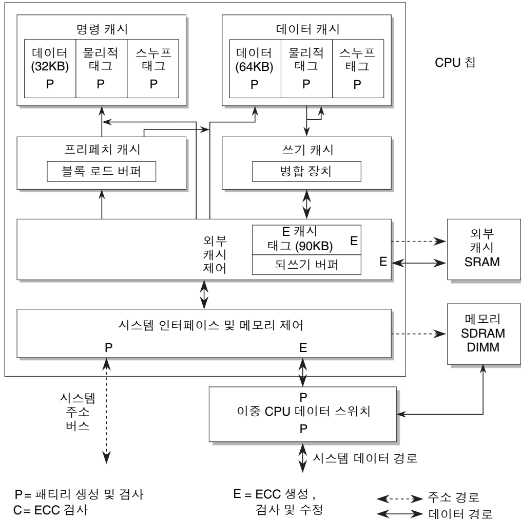
그림 3-1 CPU 오류 검출 및 수정
