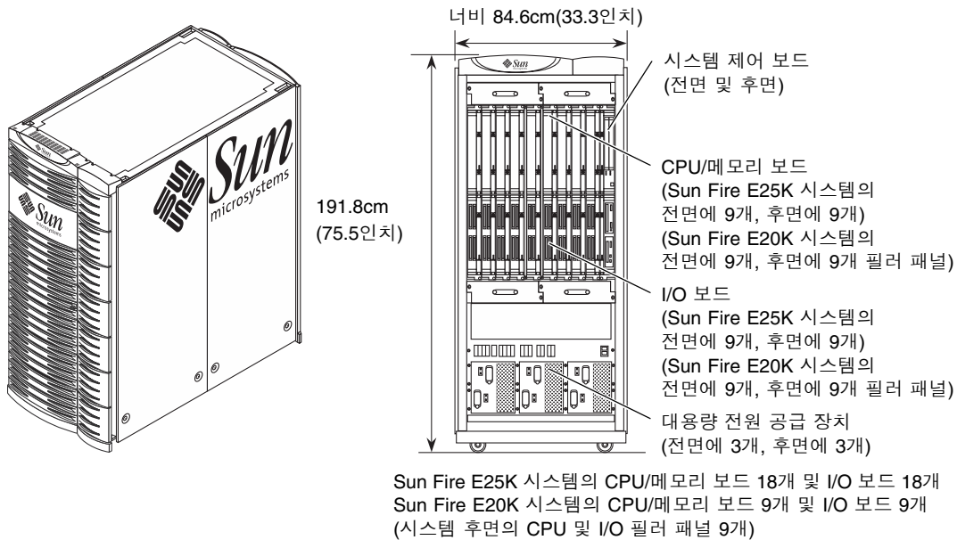
그림 1-1 Sun Fire E25K/E20K 시스템
