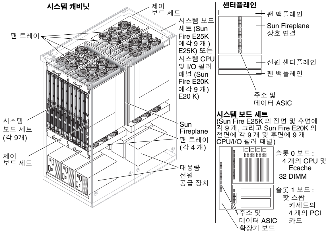
그림 5-1 Sun Fire E25K/E20K 시스템 주요 구성 요소
