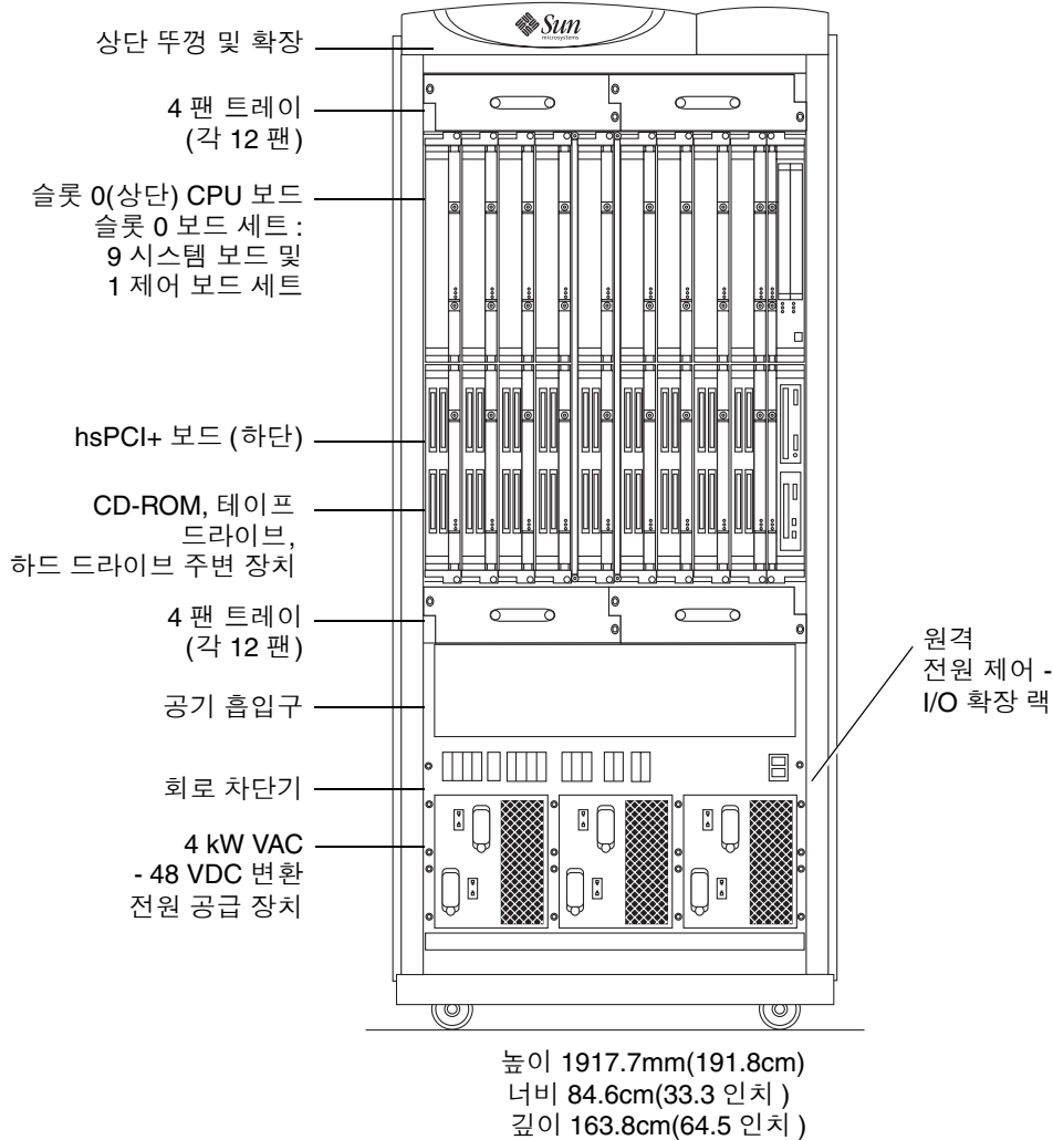
그림 5-2 Sun Fire E25K/E20K 시스템 캐비닛 — 전면
