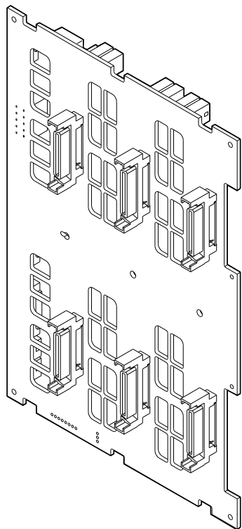
正面図
