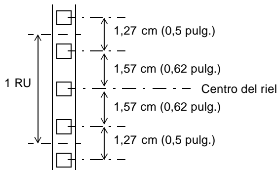
FIGURA 2-1 Dimensiones de la distribución de los orificios de montaje universal EIA/RETMA
