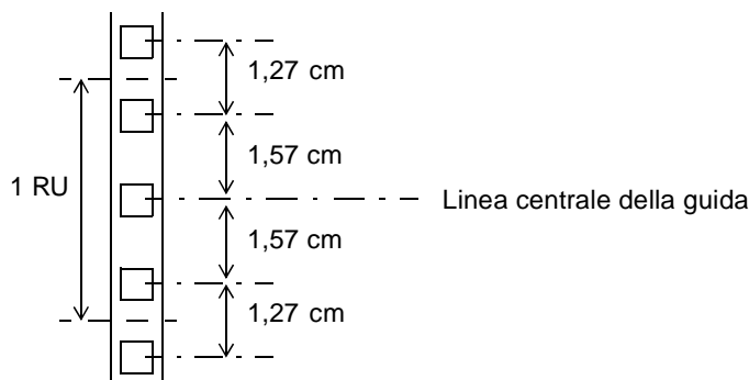
FIGURA 2-1 Dimensioni della spaziatura universale di fori EIA/RETMA per il montaggio
