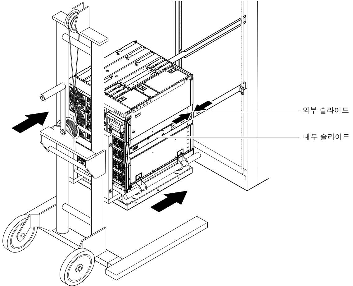
그림 1-9 슬라이드 정렬
