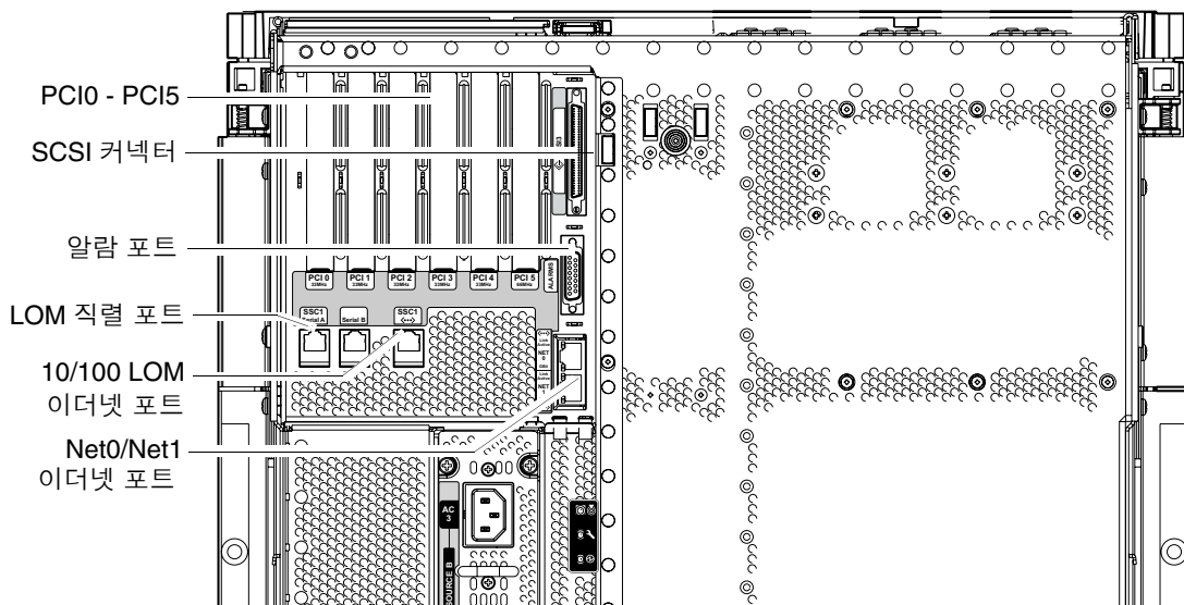
그림 A-1 외부 I/O 연결 — Sun Fire E2900 시스템(후면)
