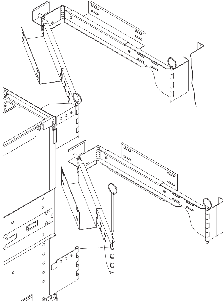
그림 1-16 상단 및 하단 케이블 암 조립
