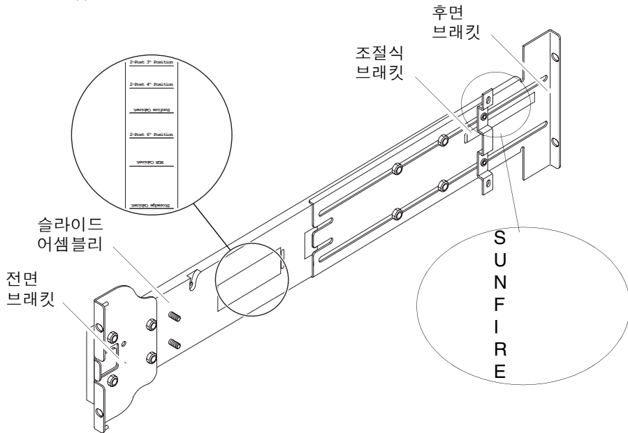
그림 1-1 레일 어셈블리(표준 구성)
