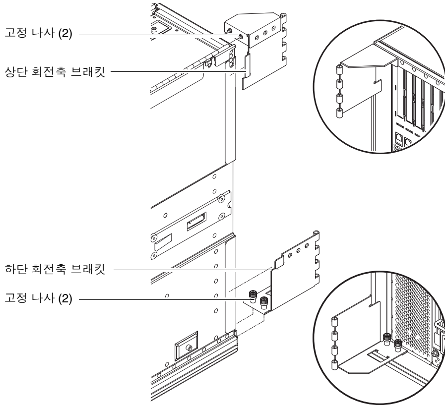
그림 1-15 상단 및 하단 회전축 브래킷 설치
