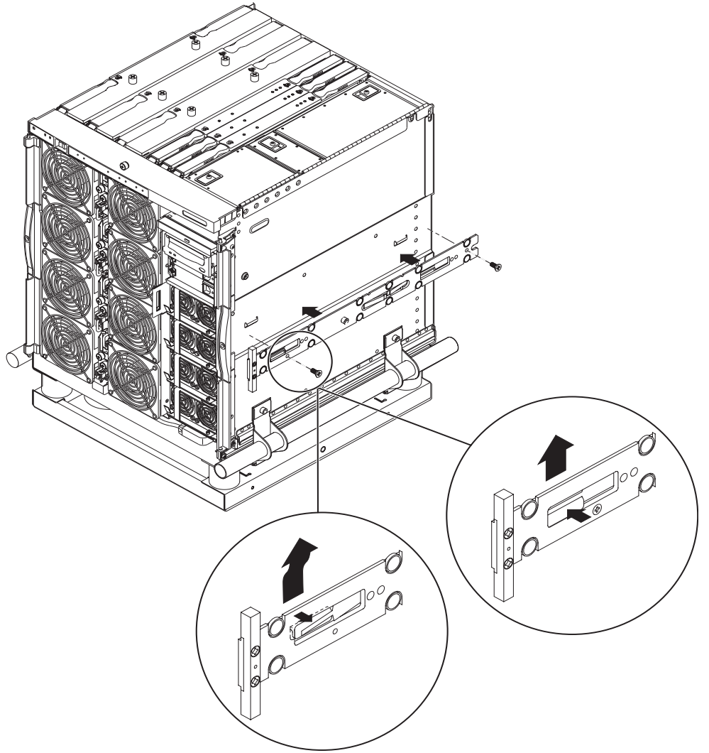
그림 1-3 스프링 클립 및 홈
