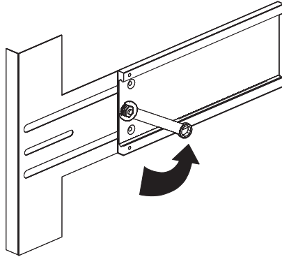
그림 1-17 슬라이드 리텐션 너트 제거
