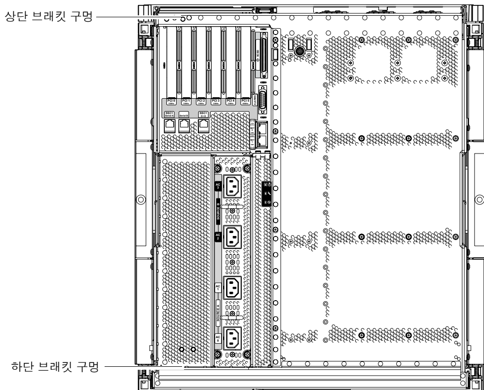
그림 1-13 브래킷 마운팅 구멍
