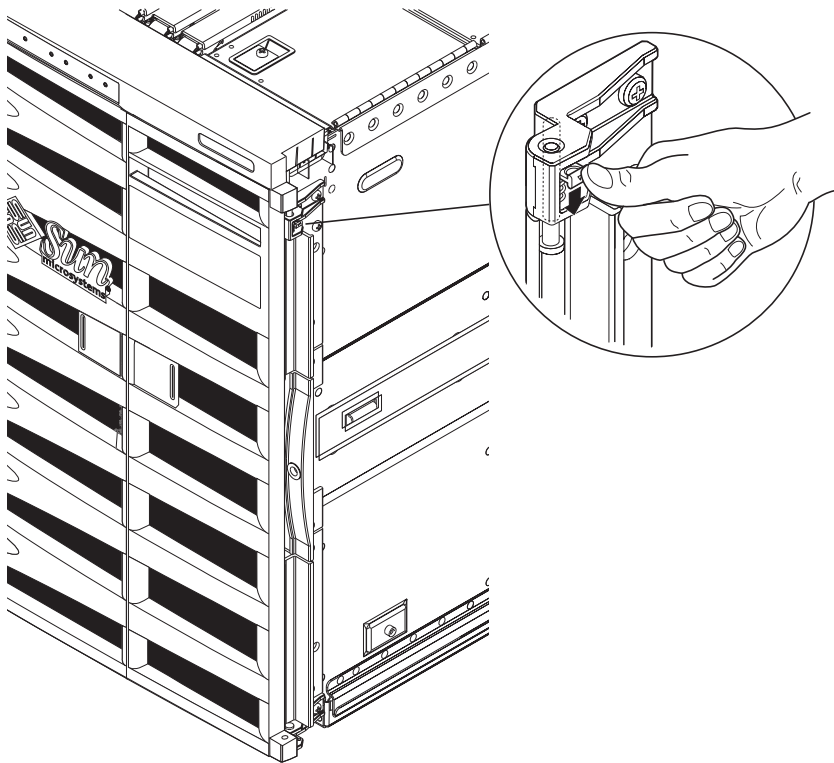
그림 1-6 문 경첩 분리 방법
