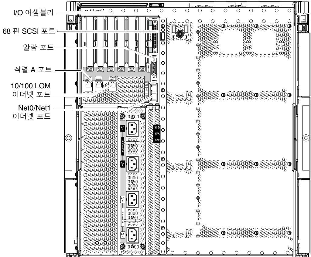
그림 1-18 시스템 컨트롤러 및 I/O 어셈블리 위치
