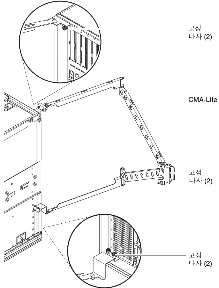
그림 1-14 CMA-Lite 케이블 관리 암
