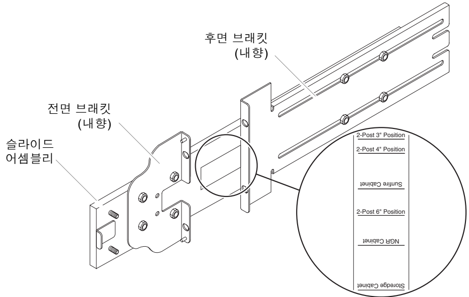
그림 1-2 레일 어셈블리(2-포스트 설치용으로 수정됨)
