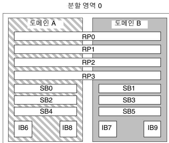
그림 1-1 단일 분할 영역 모드의 Sun Fire E6900 및 6800 시스템
