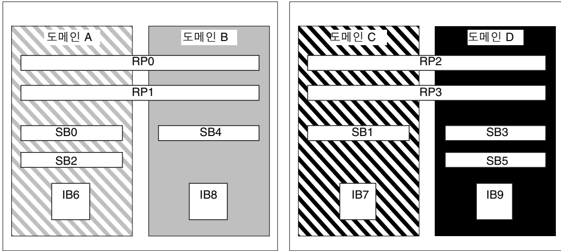
그림 1-2 이중 분할 영역 모드의 Sun Fire E6900 및 6800 시스템
