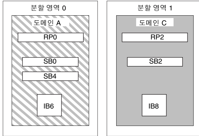
그림 1-4 이중 분할 영역 모드의 Sun Fire E4900/4810/4800 시스템
