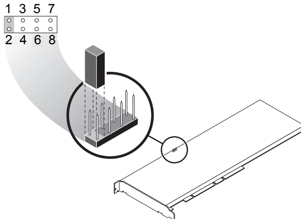
圖 G-1 硬體跳線帽針腳
