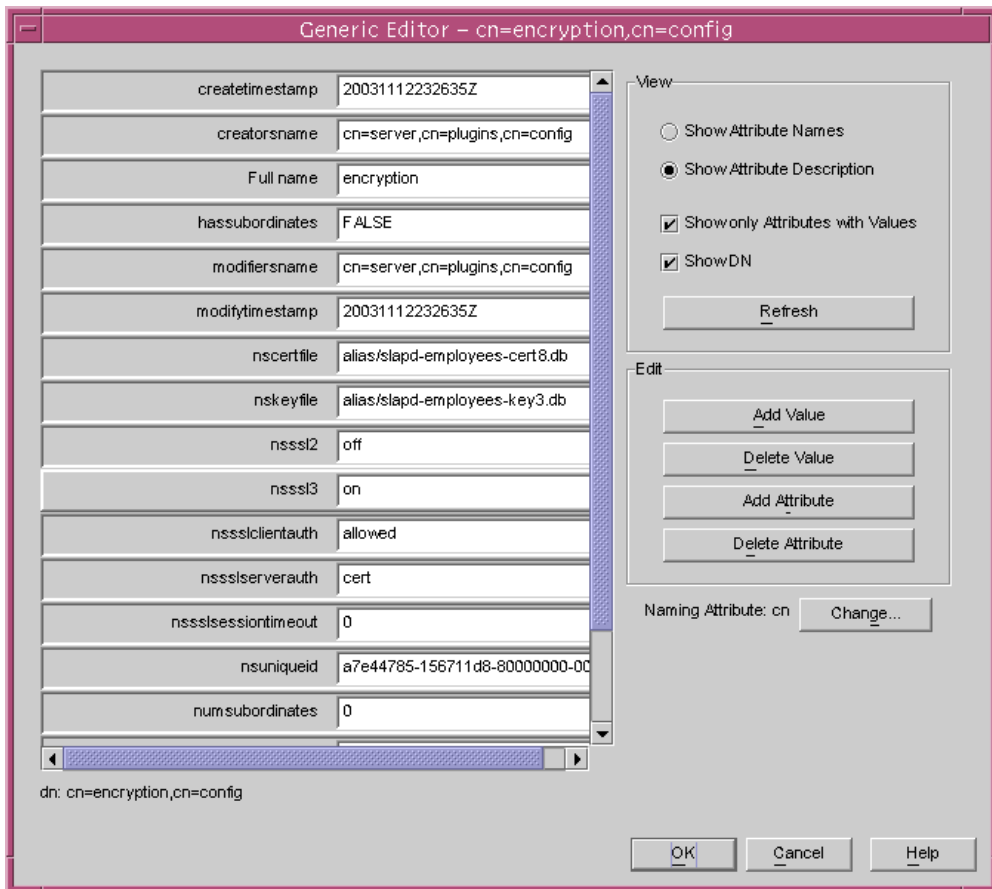
図 5-13 Sun ONE ディレクトリサーバーの cn=encryption,cn=config のダイアログボックス
