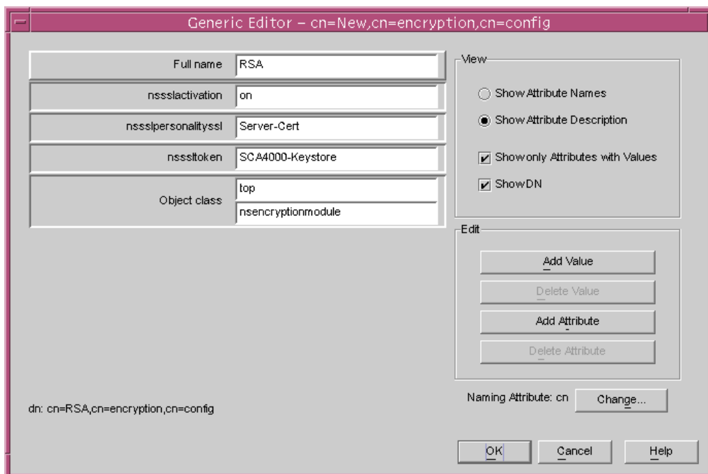
図 5-14 Sun ONE ディレクトリサーバーの nsEncryption モジュールのダイアログボックス
