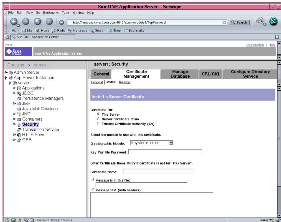
図 5-7 Sun ONE アプリケーションサーバーの管理サーバーの「Install a Server Certificate」ダイアログボックス
