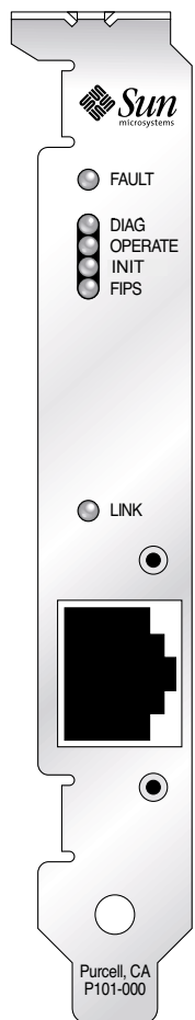
図 A-2 Sun Crypto Accelerator 4000 UTP アダプタのコネクタ
