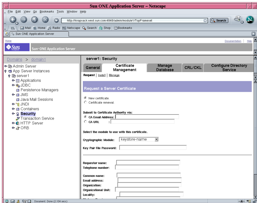
図 5-6 Sun ONE アプリケーションサーバーの管理サーバーの「Request a Server Certificate」ダイアログボックス
