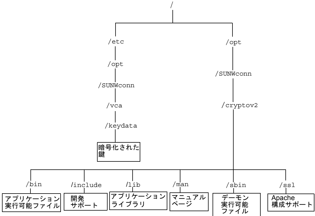
図 2-1 Sun Crypto Accelerator 4000 ディレクトリおよびファイル
