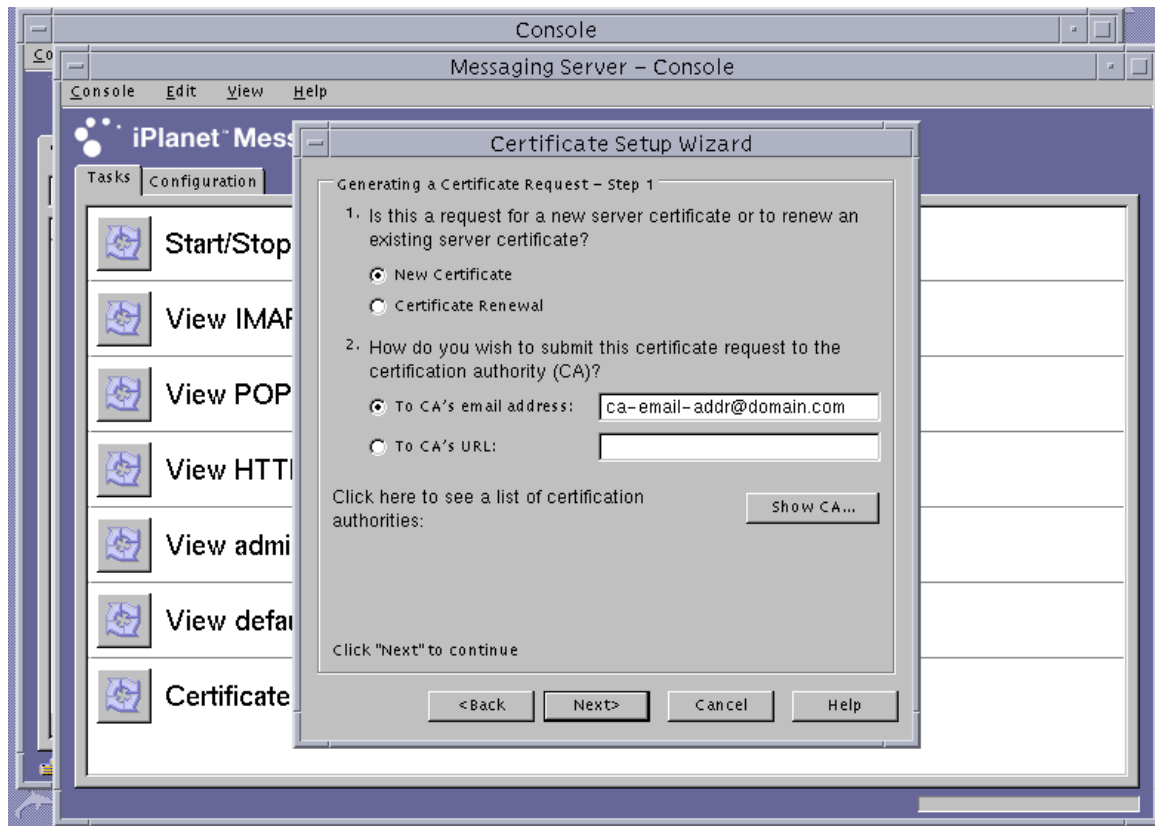
図 5-17 Sun ONE メッセージングサーバーの「Certificate Setup Wizard」の証明書要求ダイアログボックス
