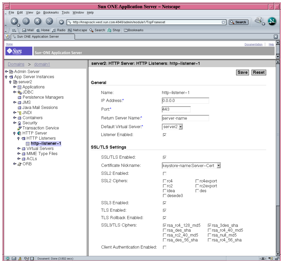
図 5-8 Sun ONE アプリケーションサーバーの管理サーバーの HTTP リスナー属性のダイアログボックス
