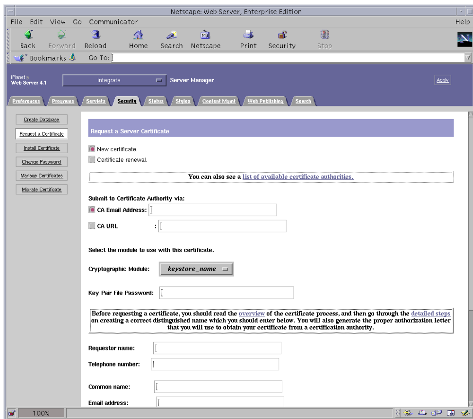
図 5-2 Sun ONE Web Server 4.1 管理サーバーの「Request a Server Certificate」ダイアログボックス
