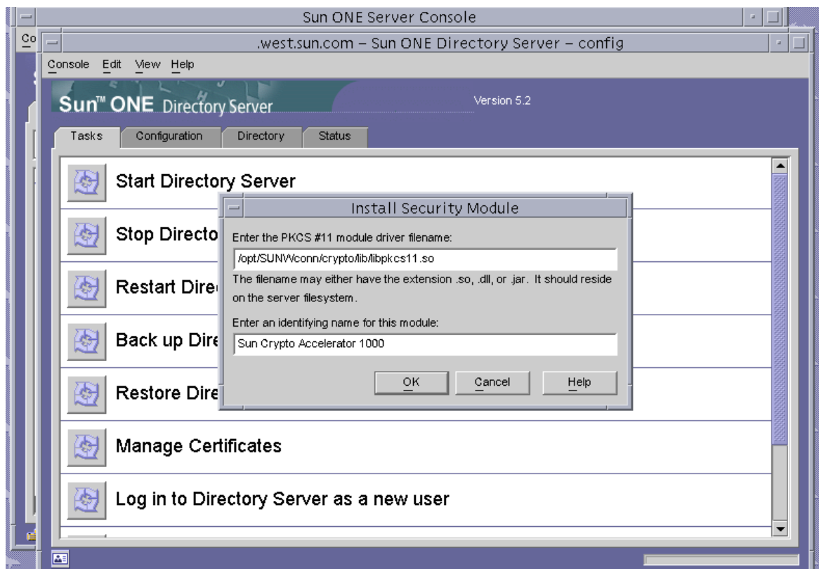
図 5-10 Sun ONE ディレクトリサーバーの「Install Security Module」ダイアログボックス
