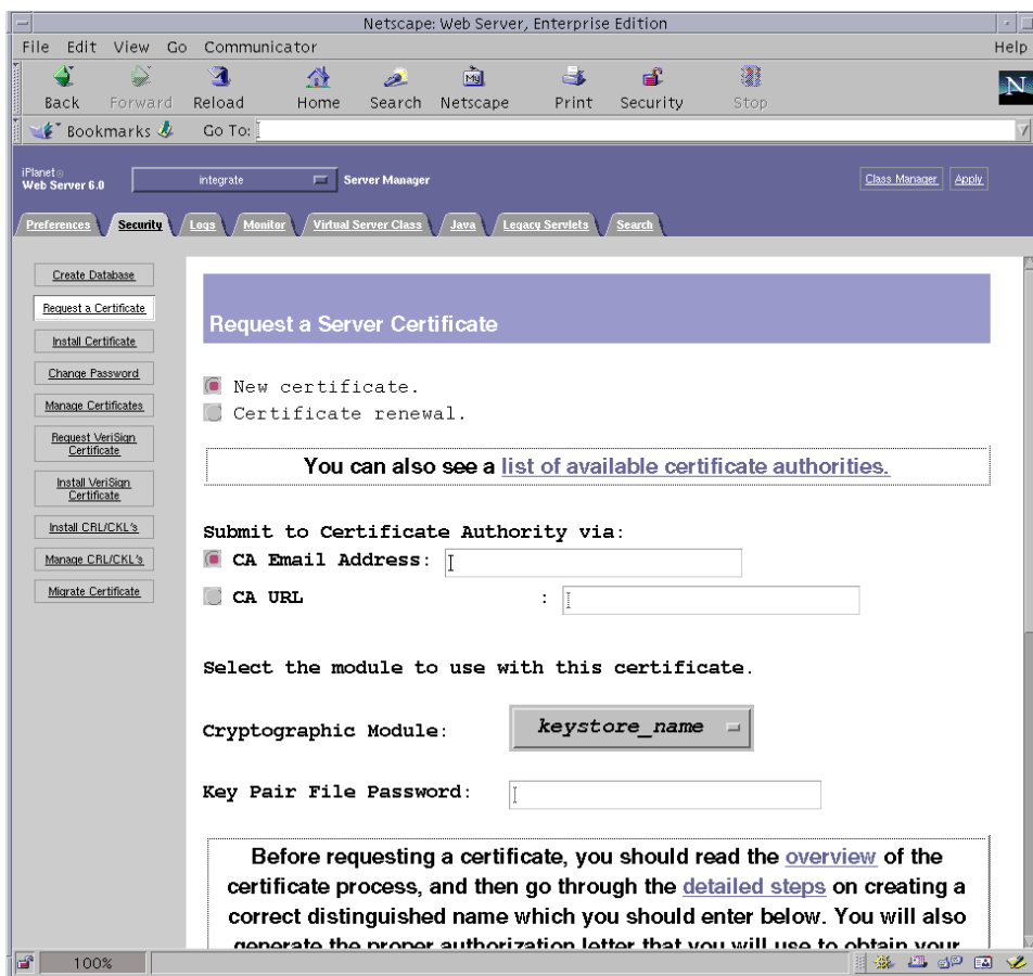
図 5-4 Sun ONE Web Server 6.0 管理サーバーの「Request a Server Certificate」ダイアログボックス
