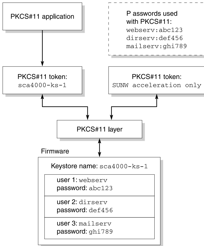
図 5-1 キーストアおよびユーザーの概要
