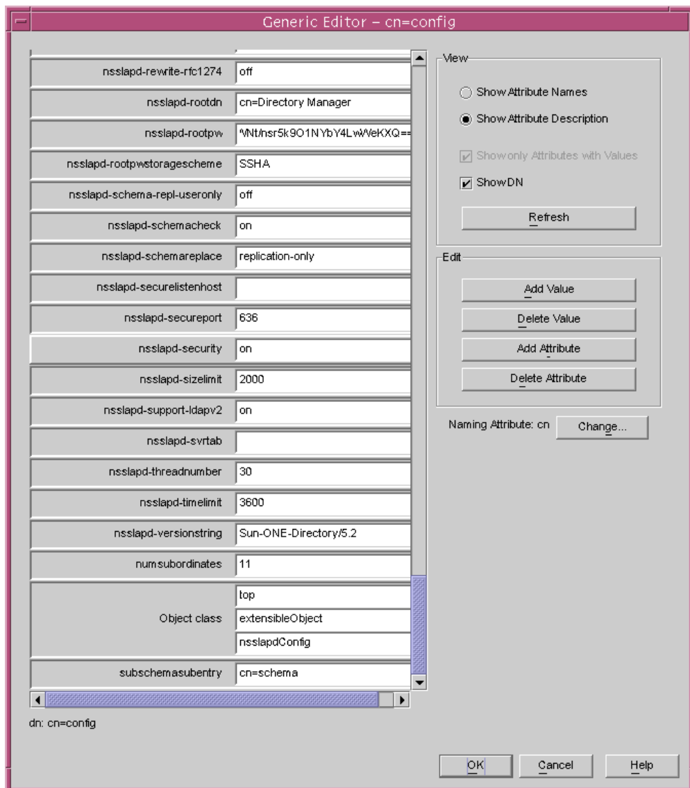
図 5-12 Sun ONE ディレクトリサーバーの cn=config の編集用ダイアログボックス
