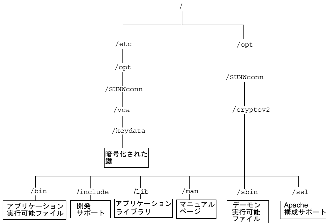
図 B-1 Sun Crypto Accelerator 4000 ディレクトリおよびファイル
