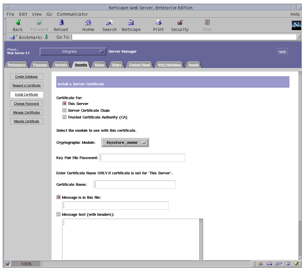
図 5-3 Sun ONE Web Server 4.1 管理サーバーの「Install a Server Certificate」ダイアログボックス
