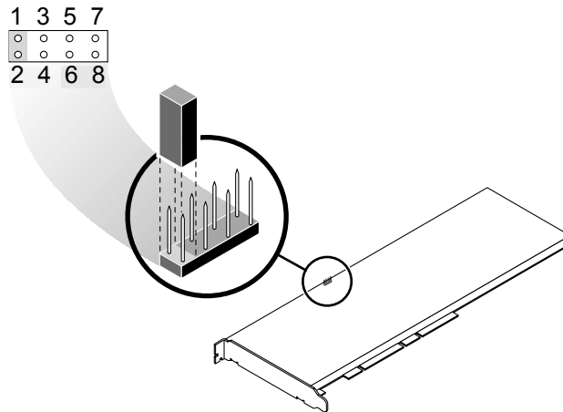
図 G-1 ハードウェアのジャンパブロックのピン
