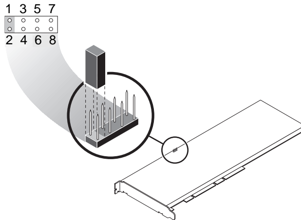
FIGURE G-1 Broches du bloc de cavaliers matériels
