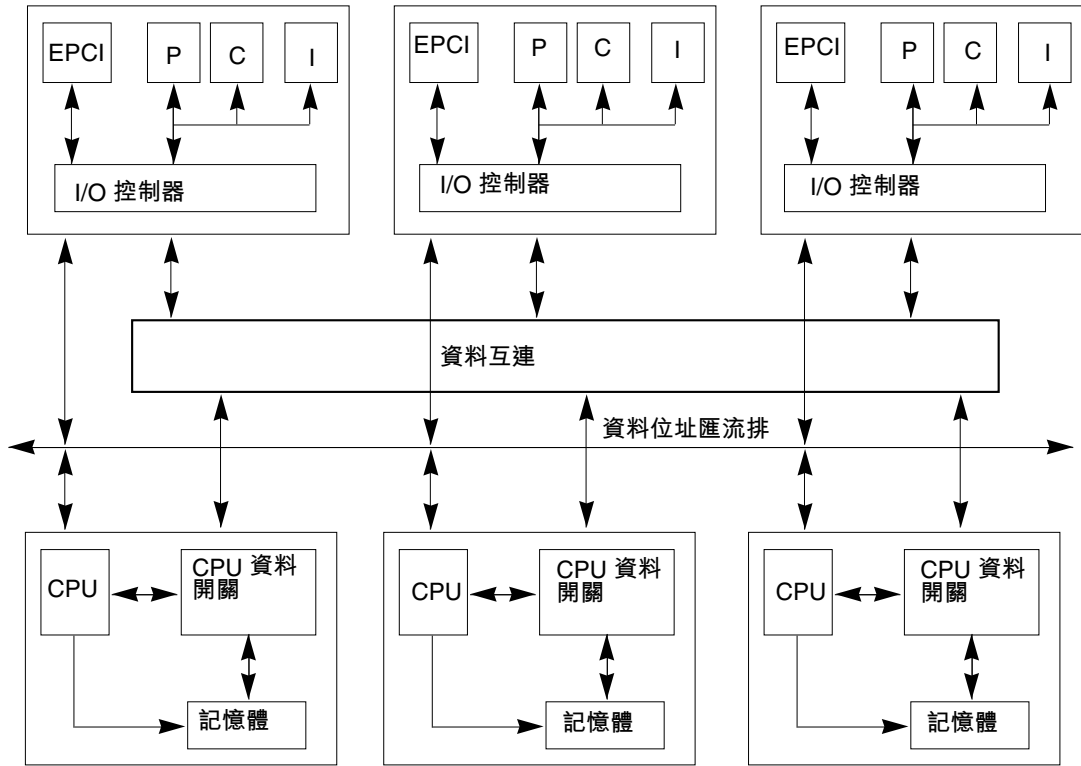
圖 3-1 Sun Fire E6900/E4900 系統的標準操作
