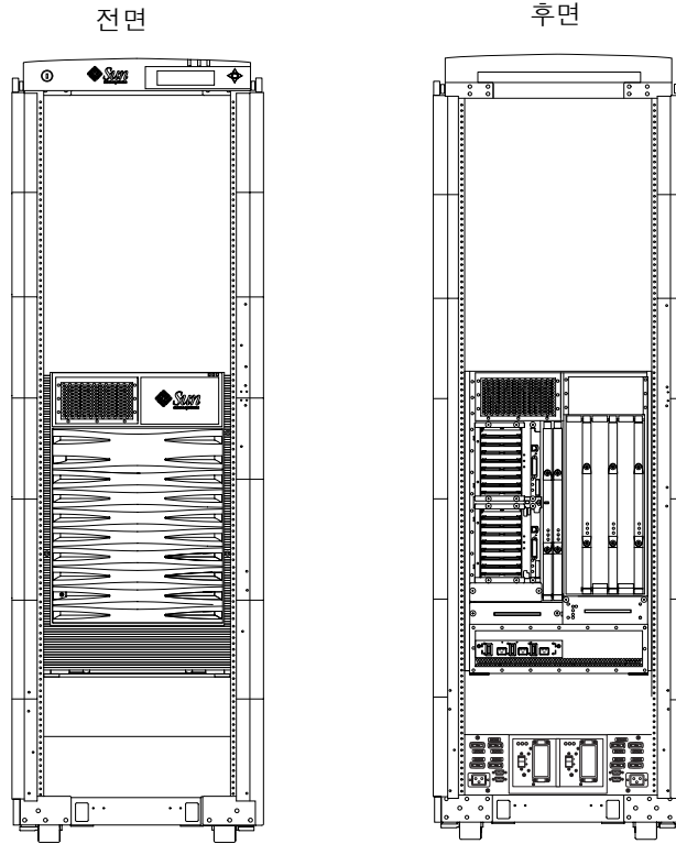
그림 2-2 Sun Fire 캐비닛 옵션에 장착된 Sun Fire E4900 시스템
