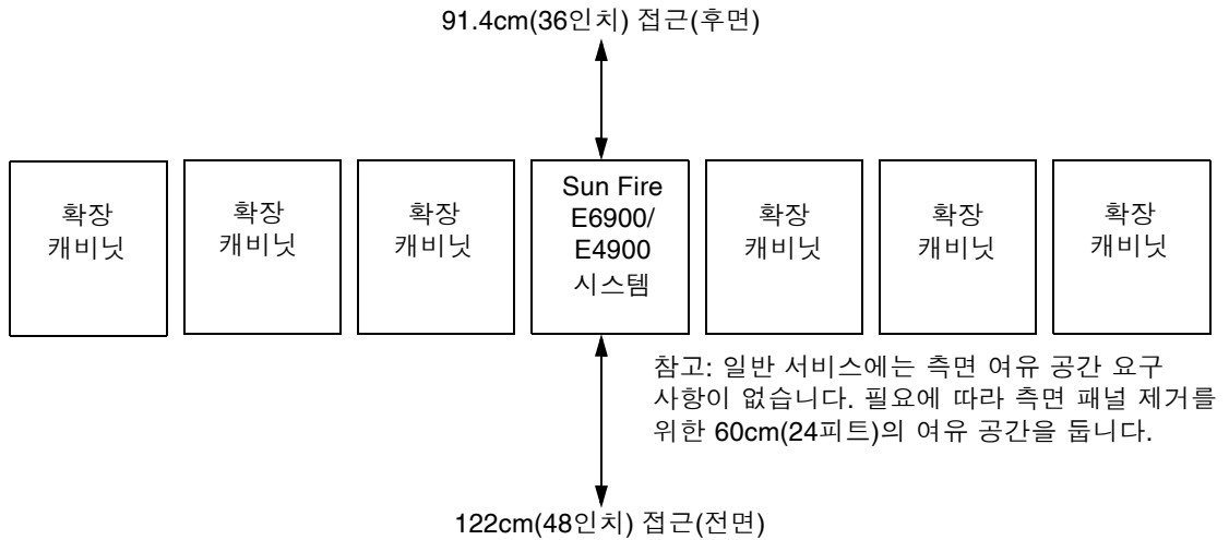
그림 2-3 Sun Fire E6900/E4900 시스템 접근 영역 — 상단 보기
