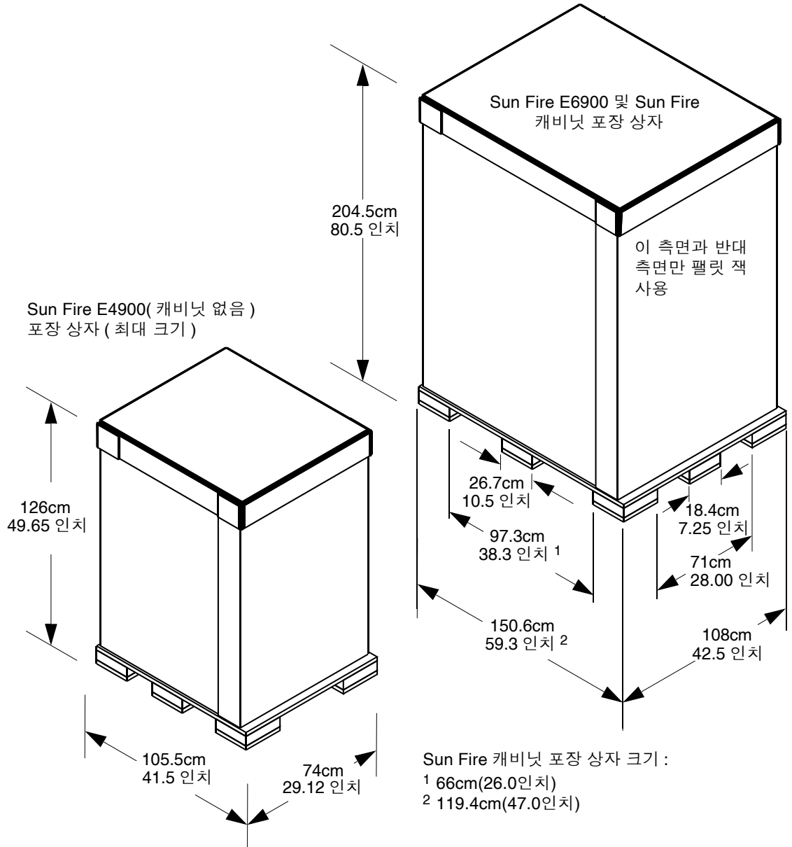
그림 2-4 포장 상자 크기
