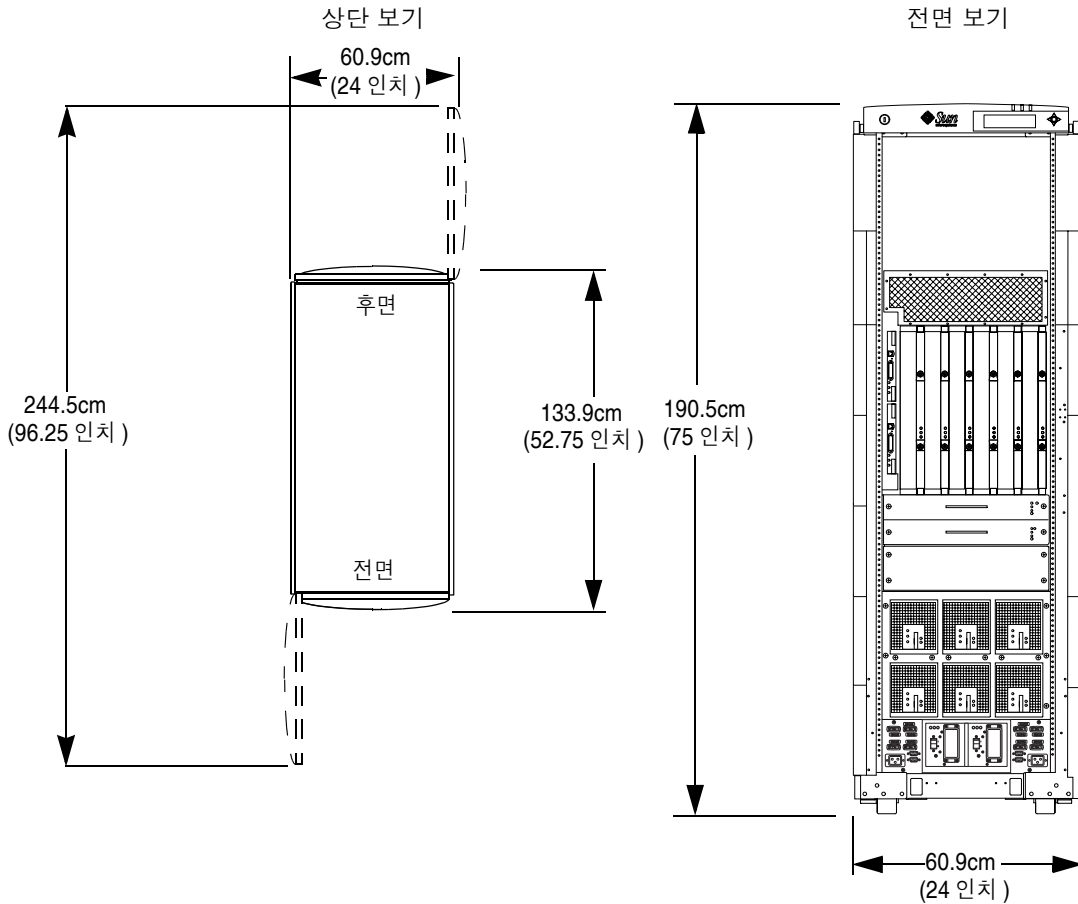
그림 2-5 Sun Fire E6900 시스템 캐비닛 크기
