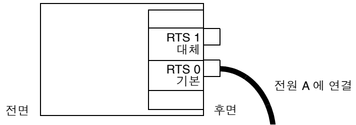
그림 3-4 1개의 RTU 어셈블리와 1개의 AC 전원
