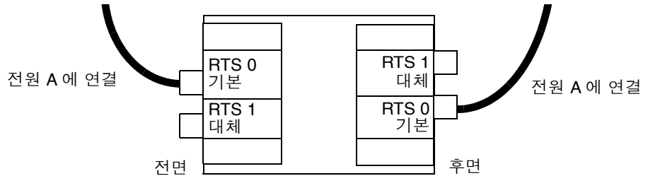
그림 3-3 2개의 RTU 어셈블리와 1개의 AC 전원
