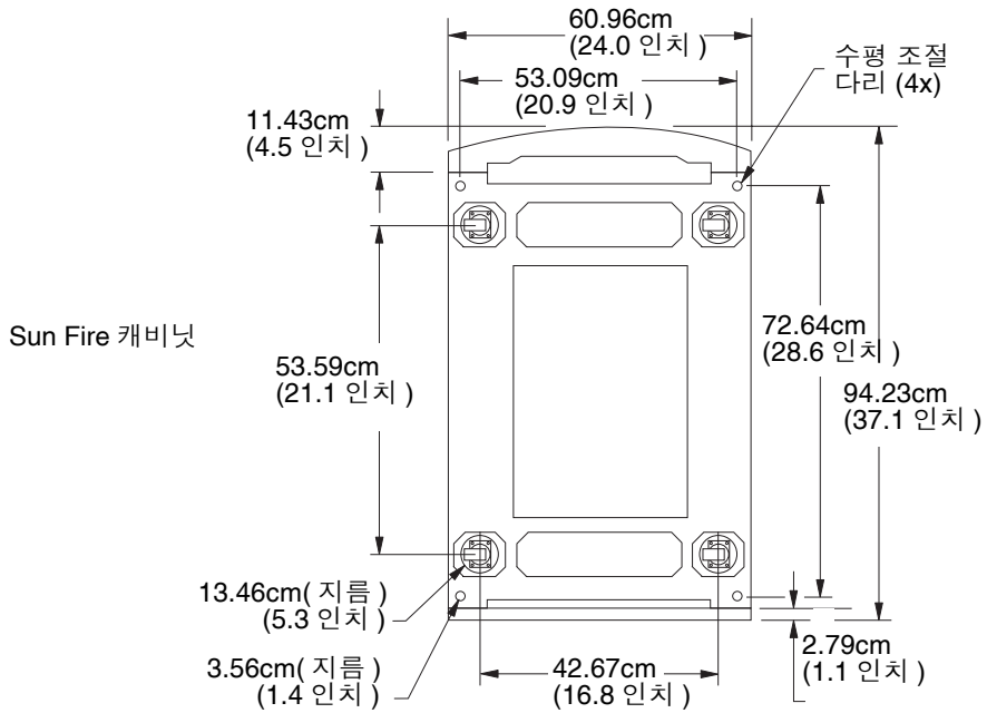
그림 2-6 Sun Fire E6900 및 Sun Fire 캐비닛 — 하단 보기
