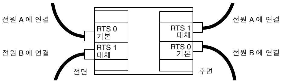
그림 3-1 2개의 RTU 어셈블리와 분리된 2개의 AC 전원
