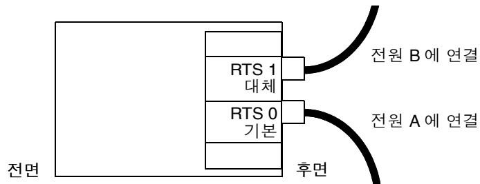
그림 3-2 1개의 RTU 어셈블리와 분리된 2개의 AC 전원
