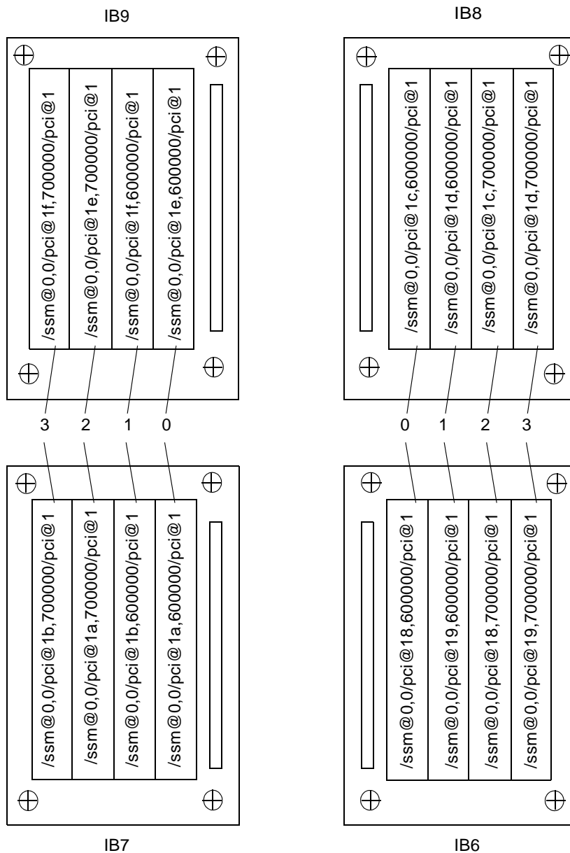
圖 A-5 Sun Fire E6900 和 6800 系統 IB6 至 IB9 的 4 插槽 CompactPCI 實體插槽指派
