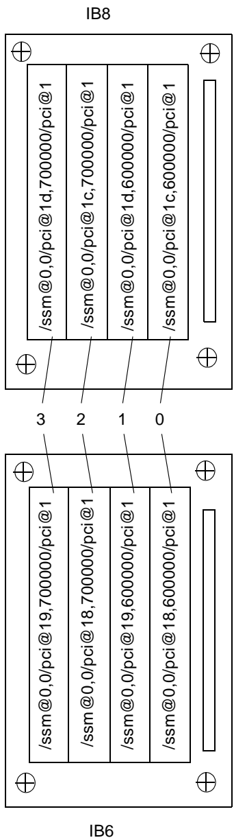
圖 A-4 Sun Fire E4900/4810/4800 系統 4 插槽 CompactPCI 實體插槽指派
