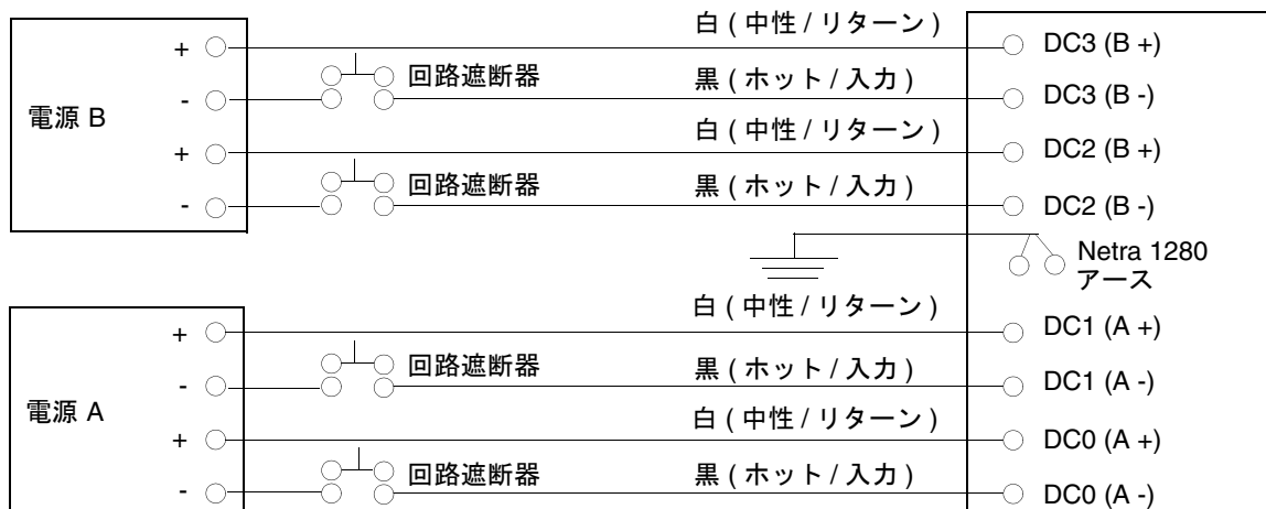
図 1-22 Netra 1280 の電力供給線のコネクタ
