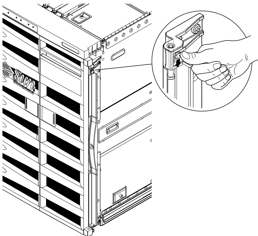
図 1-8 ドアのヒンジの外し方
