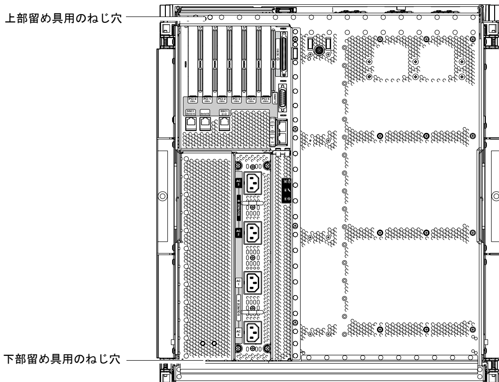
図 1-17 留め具の取り付け用ねじ穴
