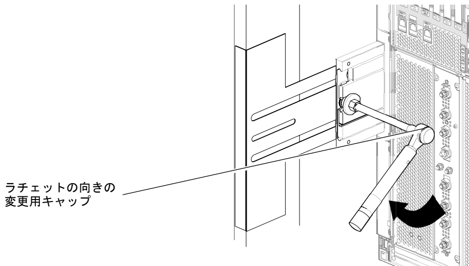
図 1-16 トルクレンチを使用したスライドのロックナットの固定
