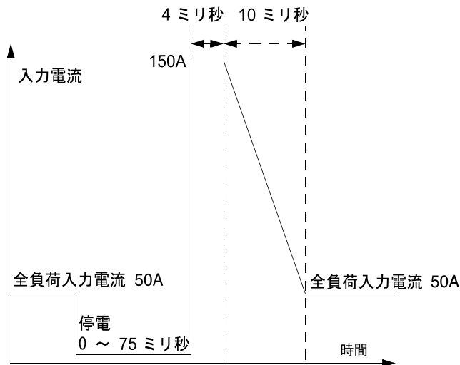
図 3-1 サージ電流
