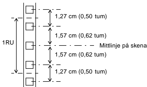
FIGUR 2-1 Universella EIA/RETMA-mått för monteringshål
