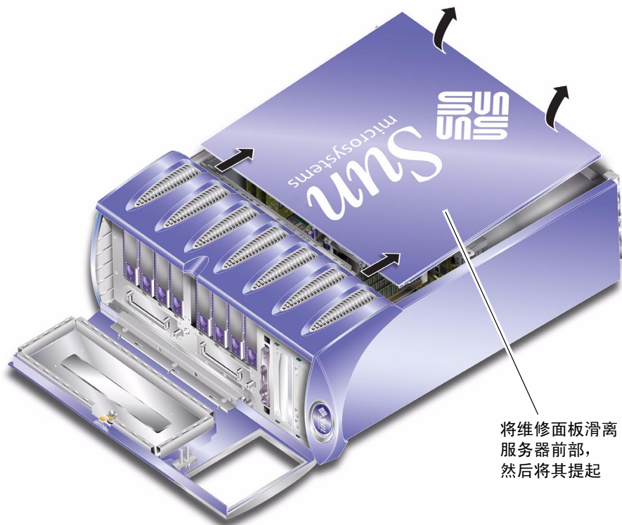
图 1-4 拆卸维修面板
