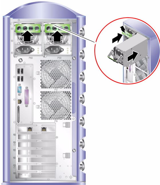
图 1-9 装回电源设备
