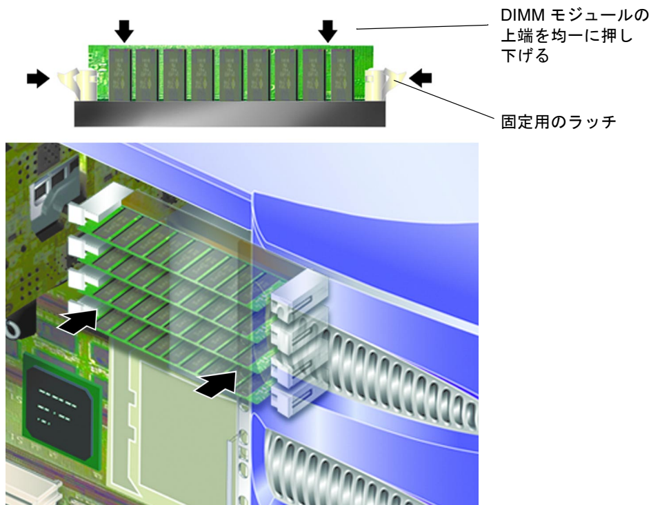
図 1-15 DIMM の挿入
