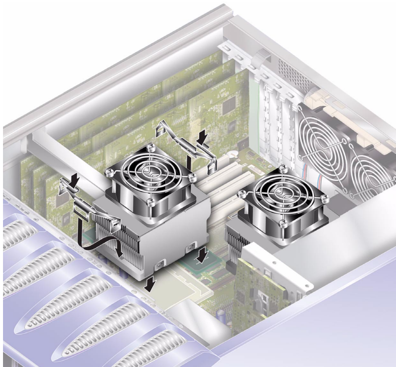
FIGURA 1-20 Sostituzione del gruppo della ventola e del dissipatore di calore del processore
