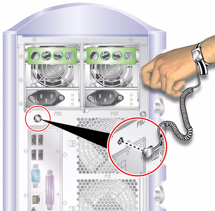
FIGURE 1-2 Point de mise à la terre du panneau arrière
