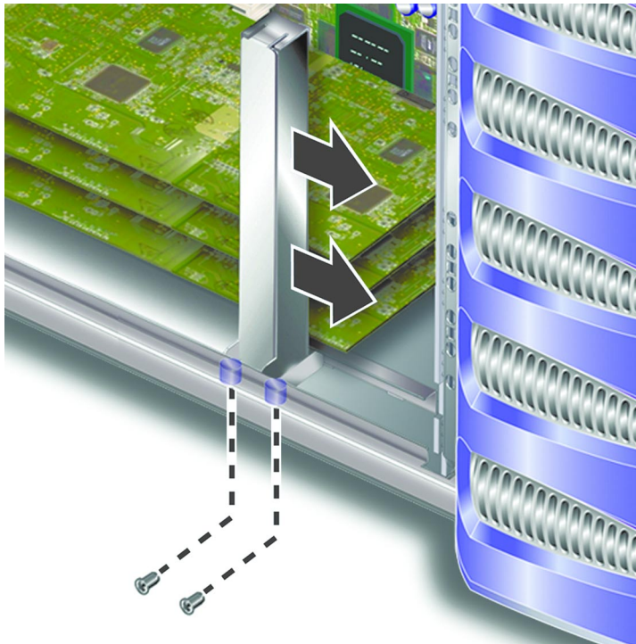
FIGURE 1-25 Déplacement du support de carte PCI longue
