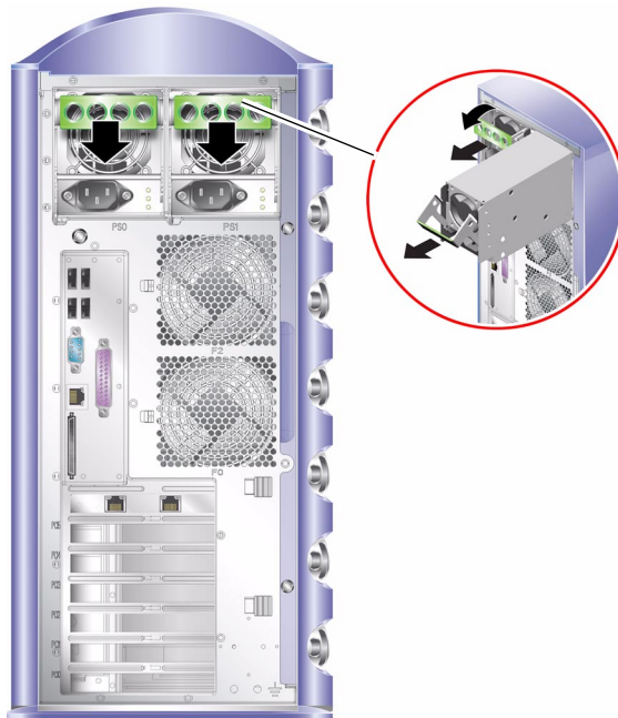
FIGURE 1-8 Retrait d'une unité d'alimentation
