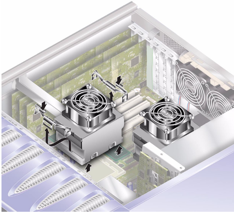
FIGURE 1-19 Retrait du ventilateur du processeur
