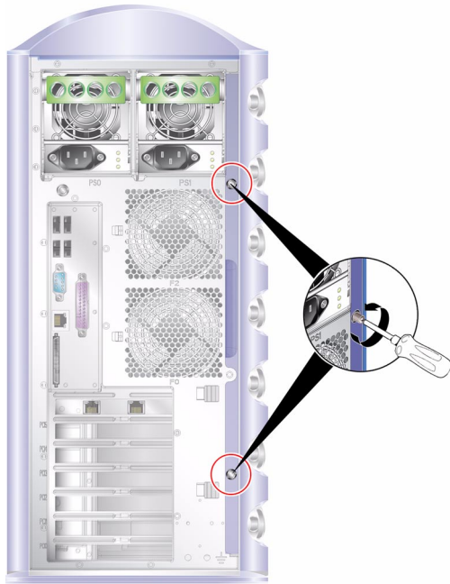
FIGURE 1-3 Emplacement des vis de retenue du panneau de service
