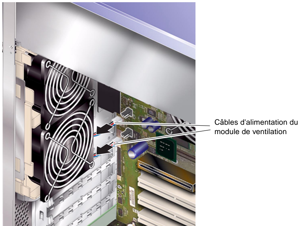
FIGURE 1-17 Déconnexion des câbles d'alimentation du module de ventilation
