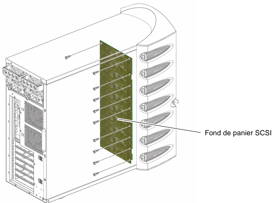
FIGURE 1-26 Emplacement du fond de panier SCSI et des vis de fixation
