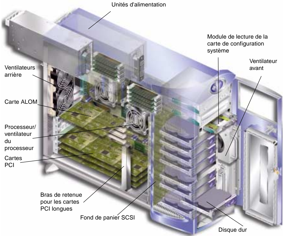
FIGURE 1-5 Emplacement des composants internes
