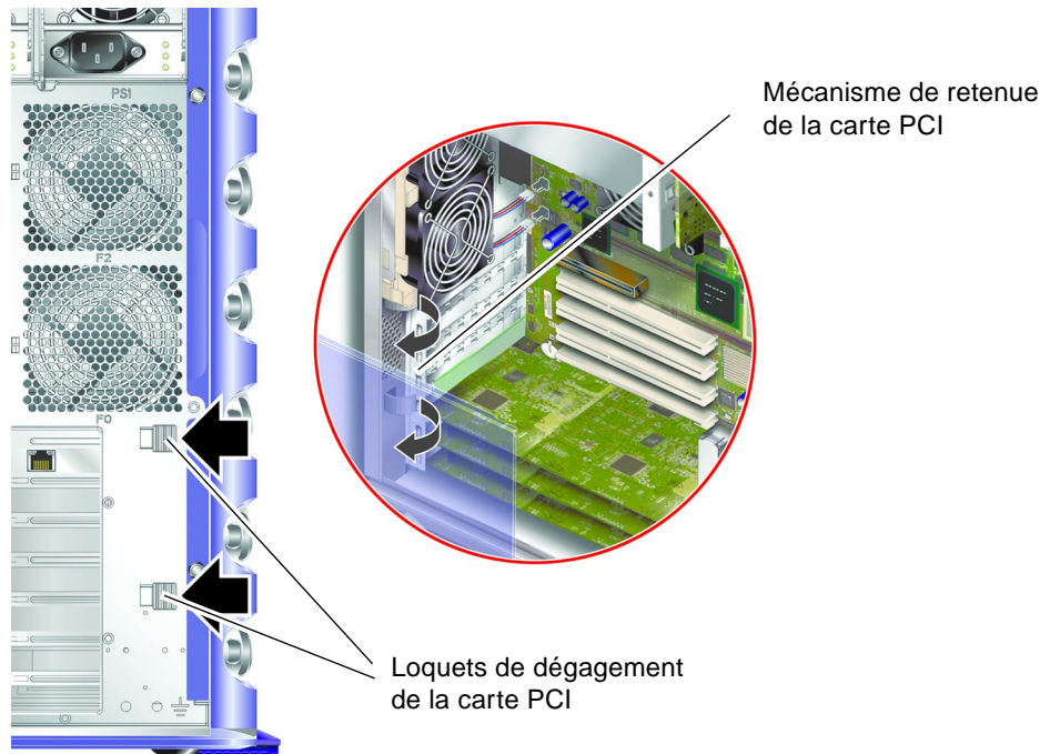
FIGURE 1-24 Mécanisme de retenue de la carte PCI
