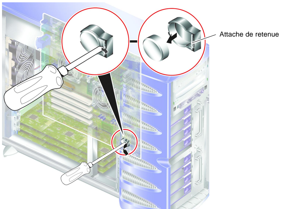
FIGURE 1-34 Retrait de la batterie
