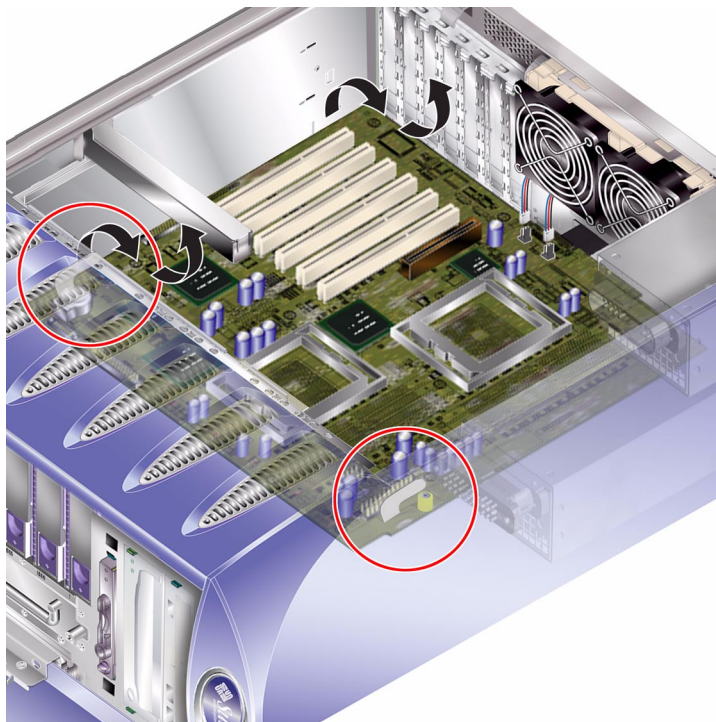
FIGURE 1-23 Retrait de la carte système du châssis
