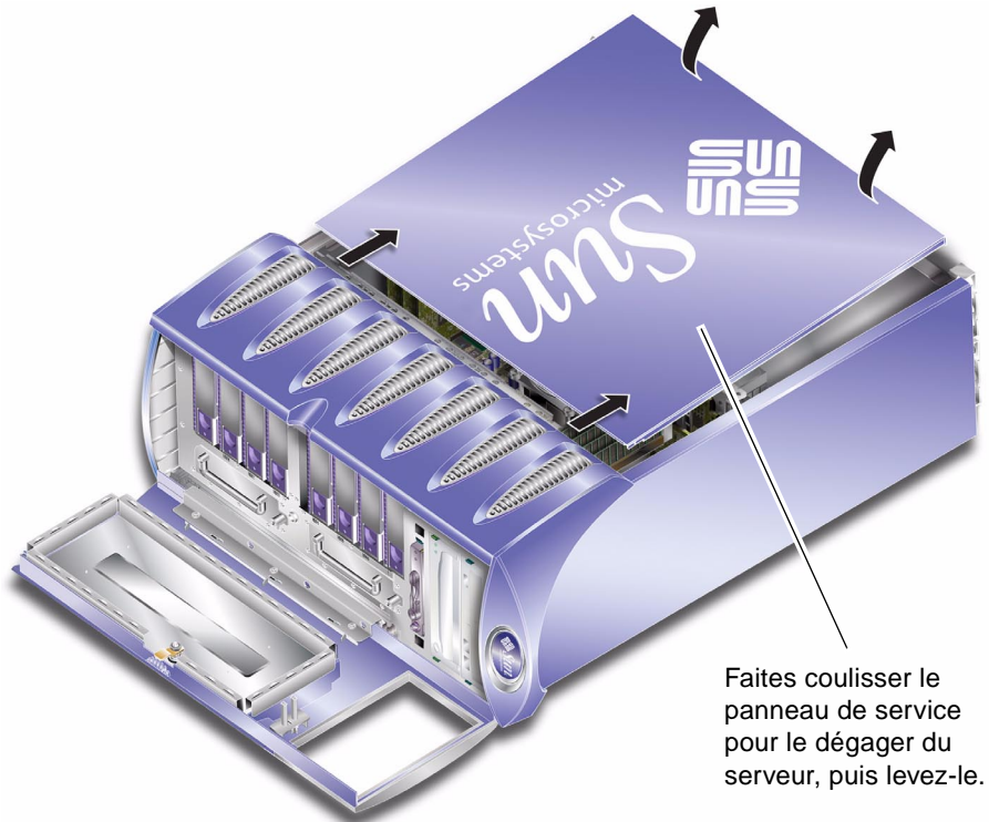
FIGURE 1-4 Retrait du panneau de service
