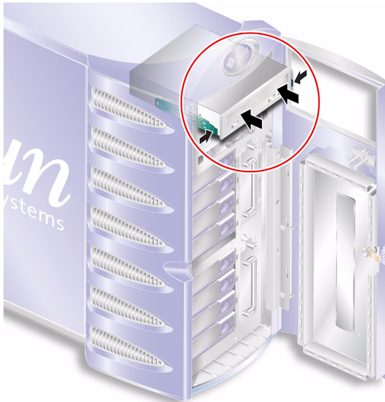
FIGURE 1-31 Réinsertion d'un lecteur de DVD-ROM
