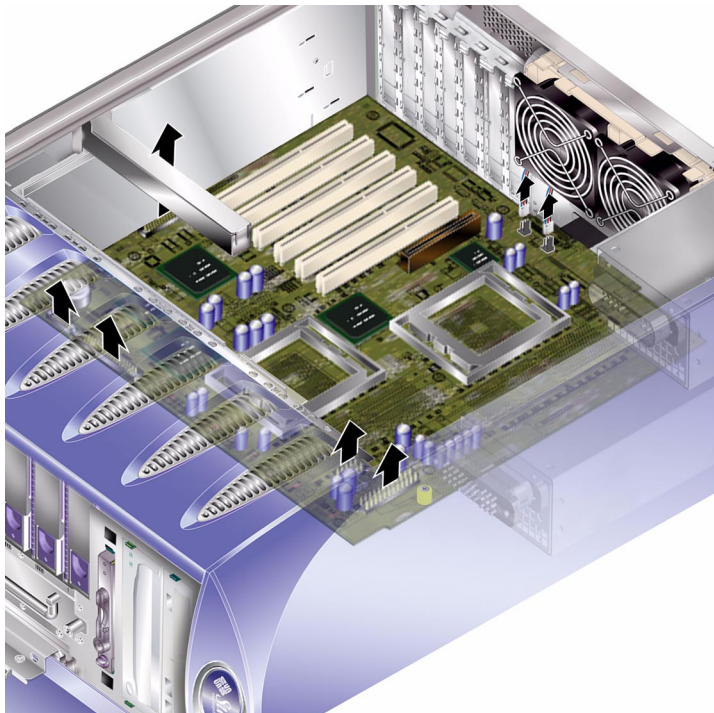
FIGURE 1-21 Retrait des câbles d'alimentation et de données de la carte système
