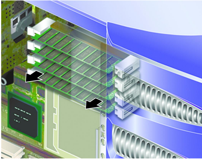
FIGURE 1-16 Retrait d'un DIMM
