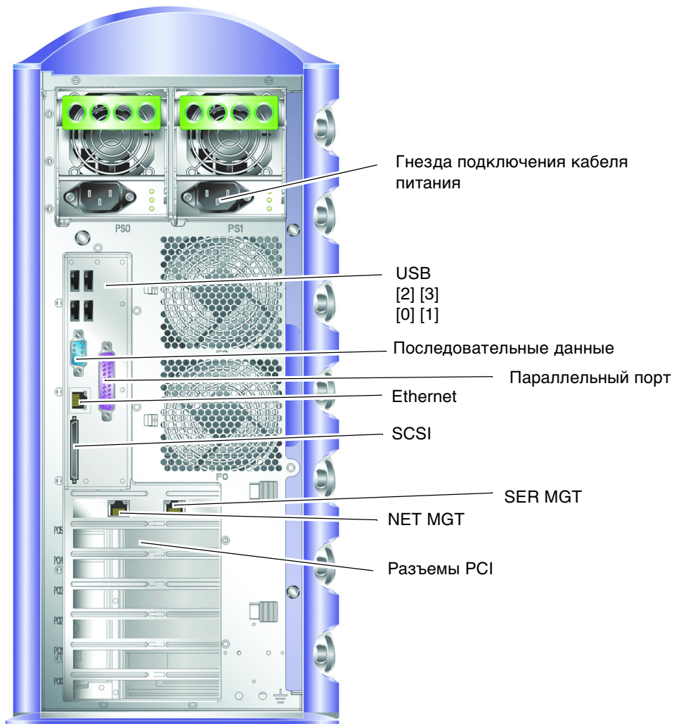
РИС. 1-4 Расположение портов ввода/вывода
