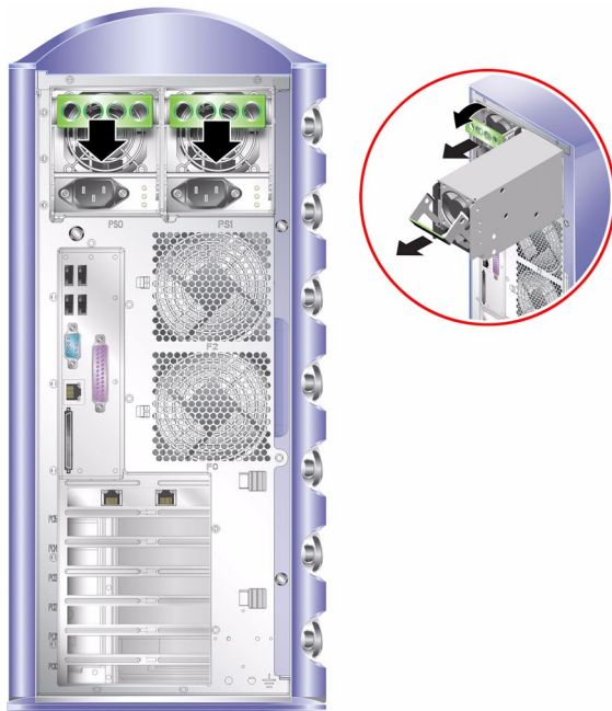
РИС. 2-4 Снятие блока питания
