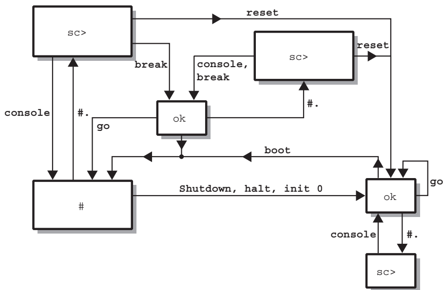
РИС. 1-5 Блок-схема приглашений системы
