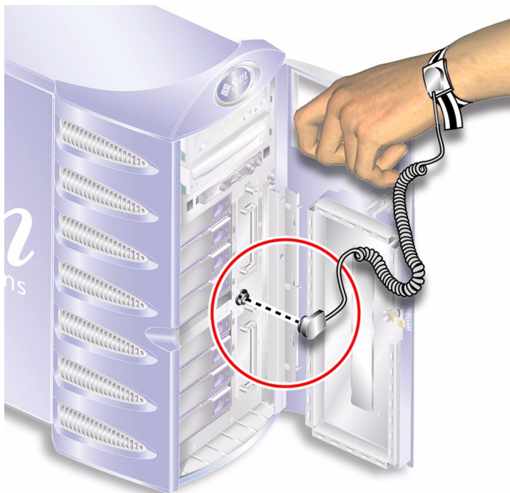
РИС. 2-1 Точка электростатического заземления на передней панели
