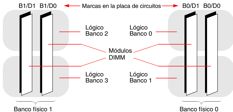
FIGURA 2-4 Cómo se asignan los bancos de memoria lógica a los módulos DIMM
