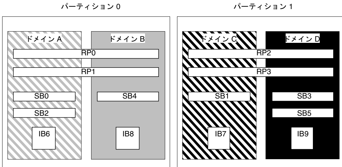
図 1-2 デュアルパーティションモードの Sun Fire 6800 システム
