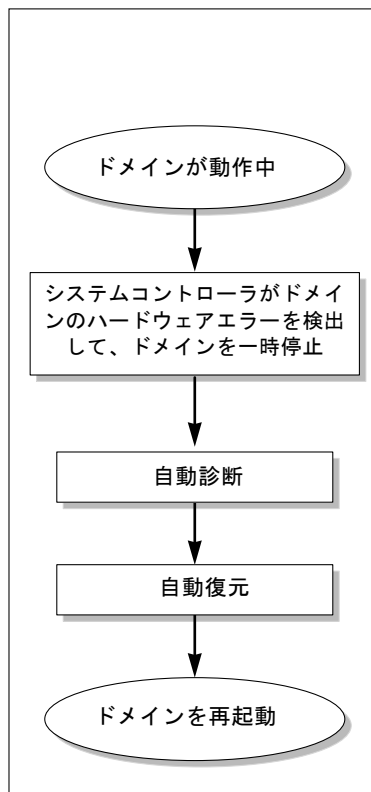
図 7-1 エラー診断およびドメイン復元処理
