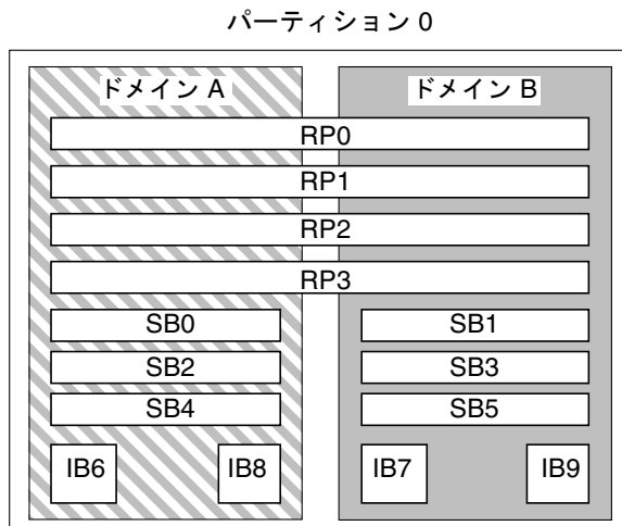
図 1-1 シングルパーティションモードの Sun Fire 6800 システム
