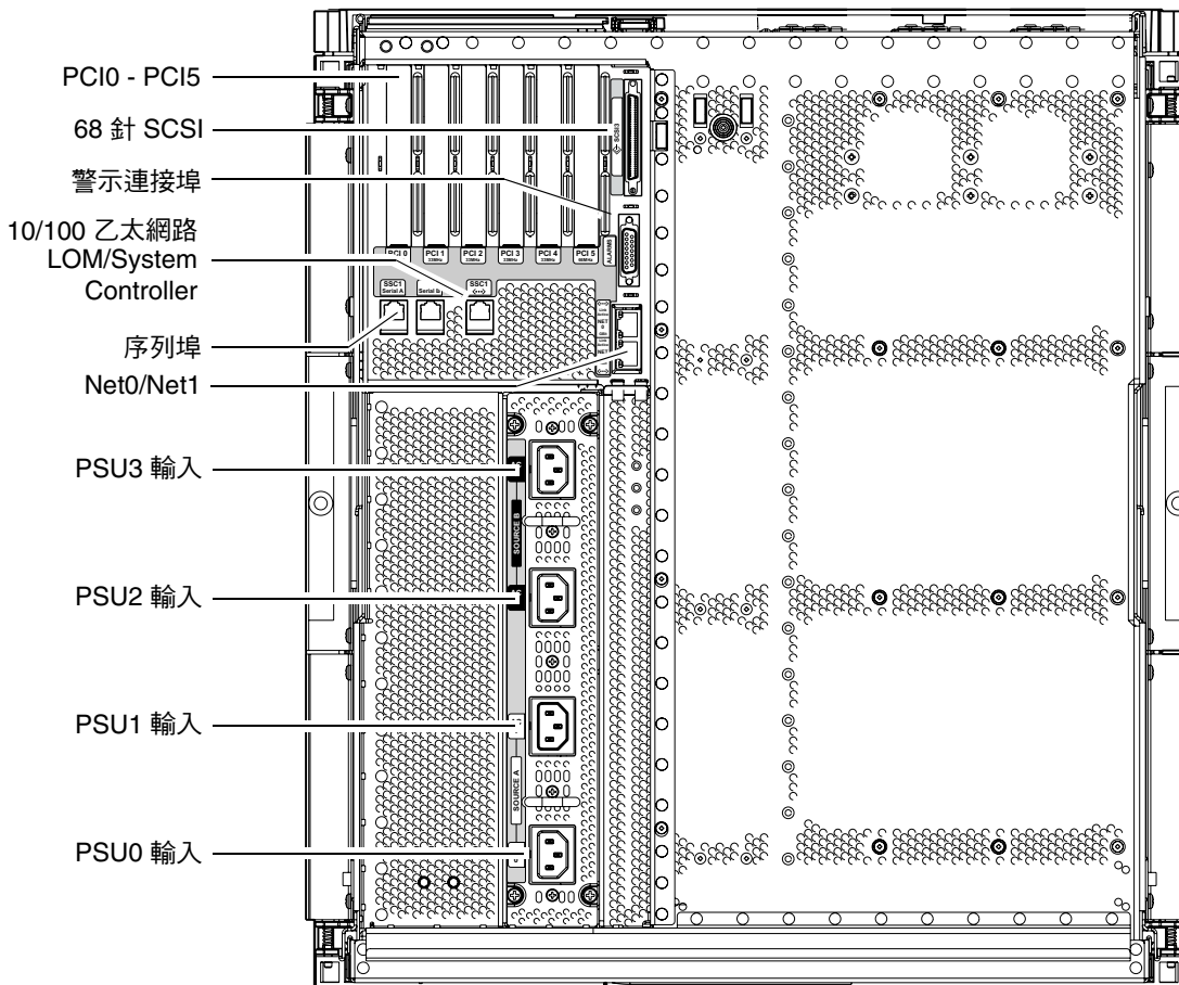
圖 1-1 I/O 連接埠
