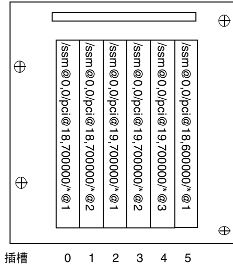
图 7-1 Sun Fire V1280/Netra 1280 IB_SSC PCI 物理插槽分配 (IB6)
