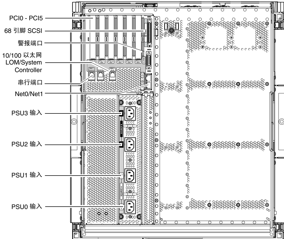
图 1-1 I/O 端口
