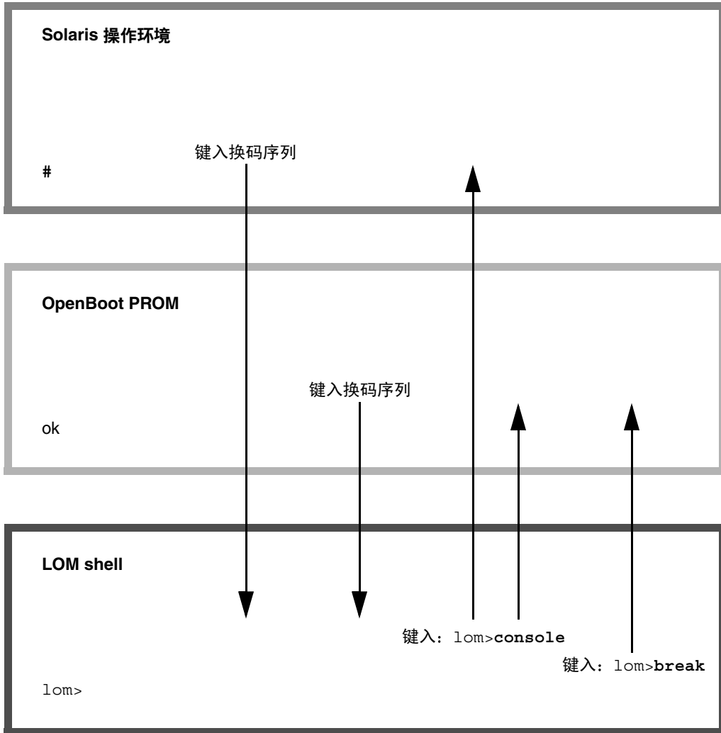
图 3-1 切换过程
