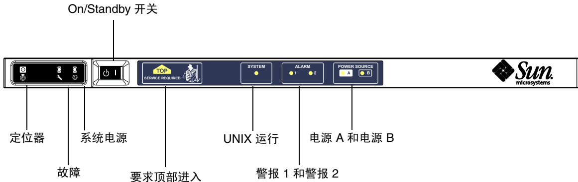
图 7-2 系统指示灯
