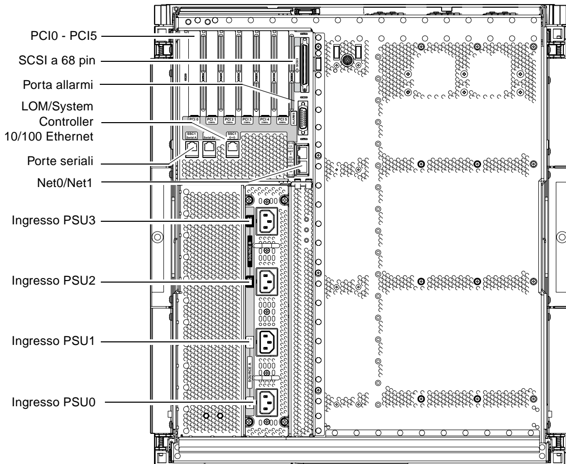
FIGURA 1-1 Porte I/O
