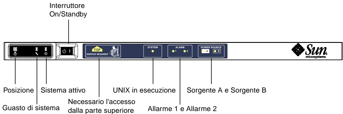
FIGURA 1-2 Scheda indicatori di sistema
