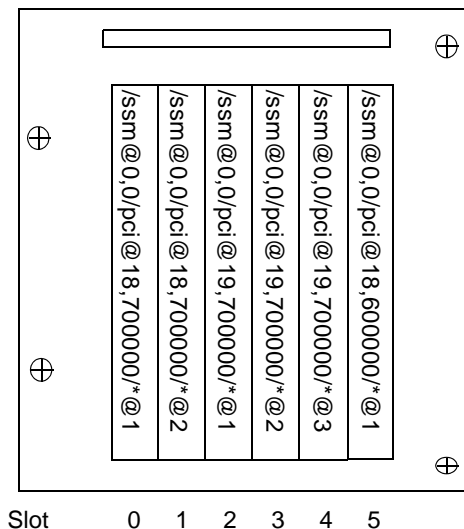
FIGURA 7-1 Designazioni di slot fisici PCI IB_SSC per IB6 nel sistema Sun Fire V1280/Netra 1280
