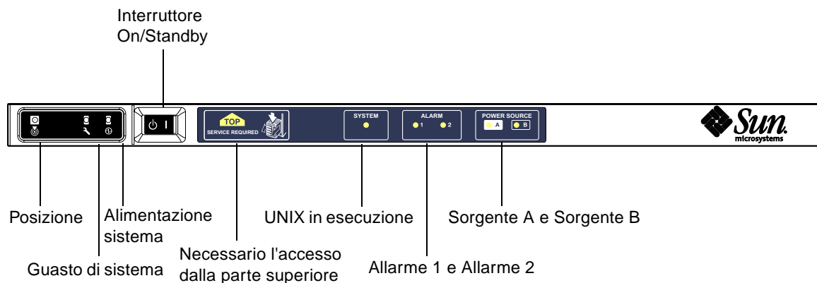
FIGURA 7-2 Indicatori di sistema
