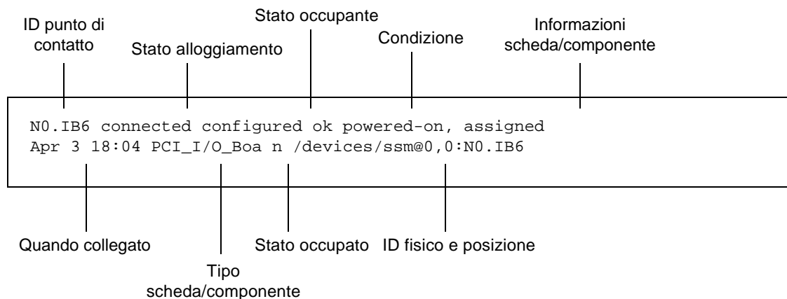
FIGURA 9-1 Dettagli della schermata per cfgadm -av
