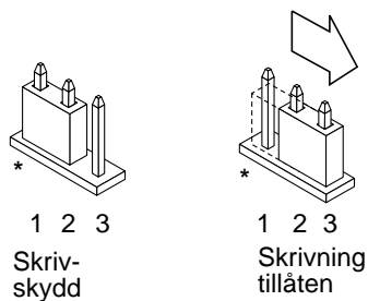
FIGUR 5-8 Ställa in bygel J3103 för skrivskydd/skrivning tillåten på Sun Enterprise 450 och Ultra 450
