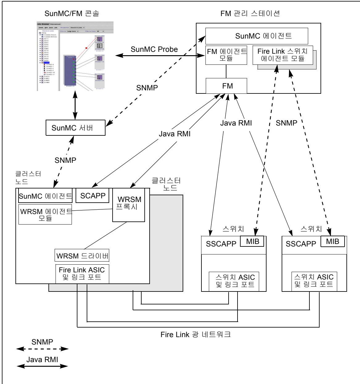
그림 1-2 Sun Fire Link 소프트웨어 구조(Sun Management Center 서버 및 콘솔 포함)
