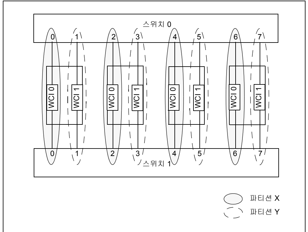
그림 6-3 이중 컨트롤러 예 - 네 개의 노드, 두 개의 스위치, 노드당 두 개의 RSM 컨트롤러
