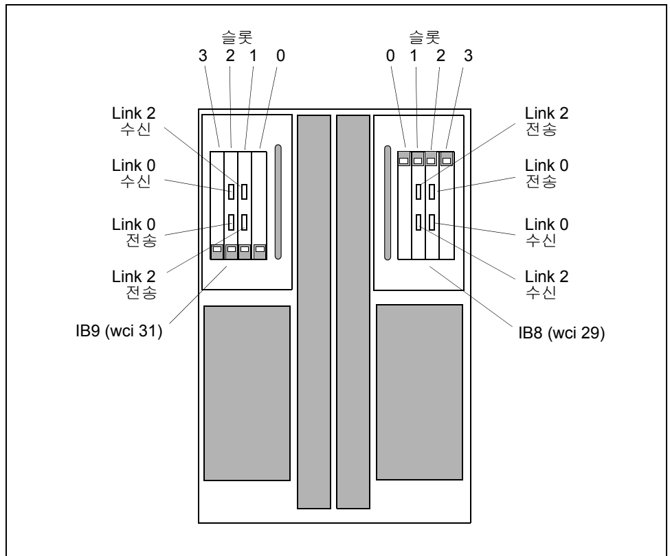
그림 10-2 Sun Fire 6800 새시에 있는 Sun Fire Link 광 포트 위치
