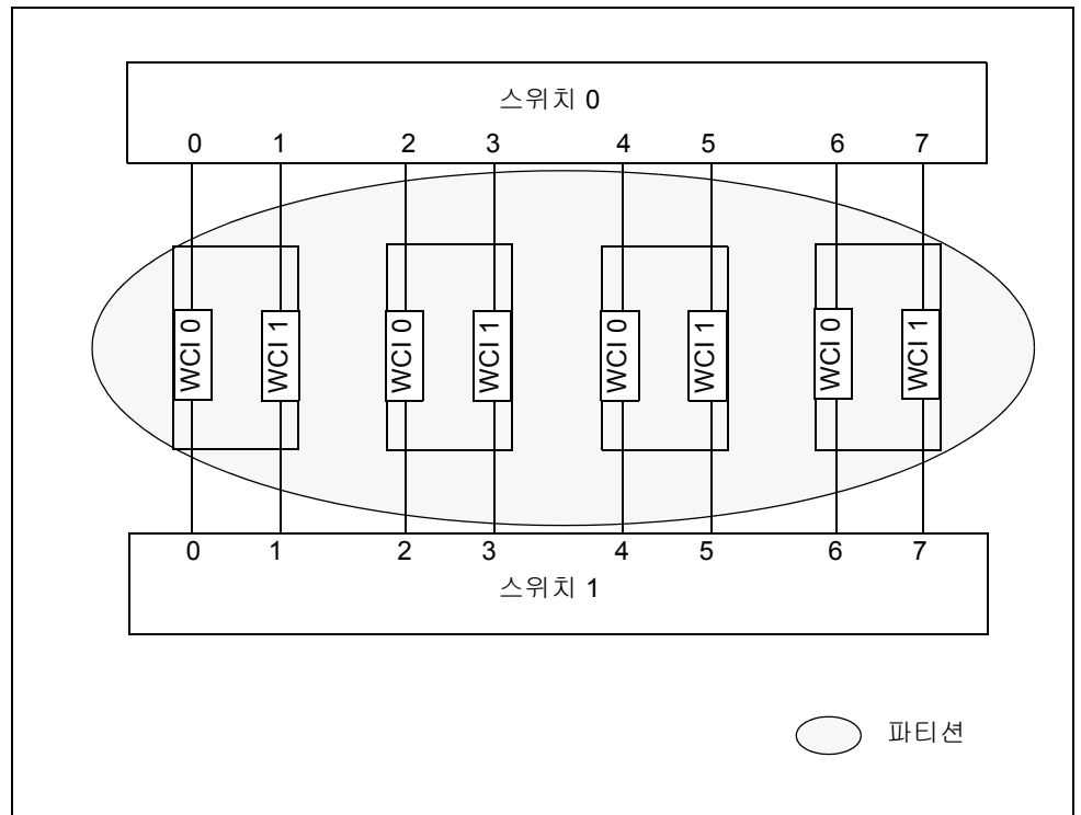
그림 6-1 단일 컨트롤러 예 - 네 개의 노드, 두 개의 스위치, 노드당 하나의 RSM 컨트롤러
