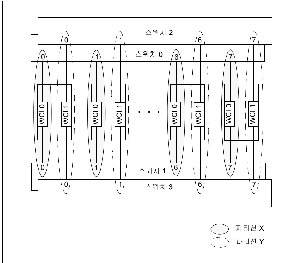
그림 6-4 이중 컨트롤러 예 - 여덟 개의 노드, 네 개의 스위치, 노드당 두 개의 RSM 컨트롤러
