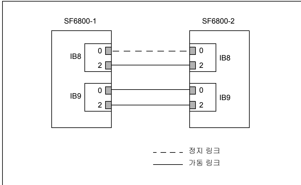
그림 10-1 하나의 정지 링크와 세 개의 가동 링크를 갖는 2 노드, 직접 연결 클러스터
