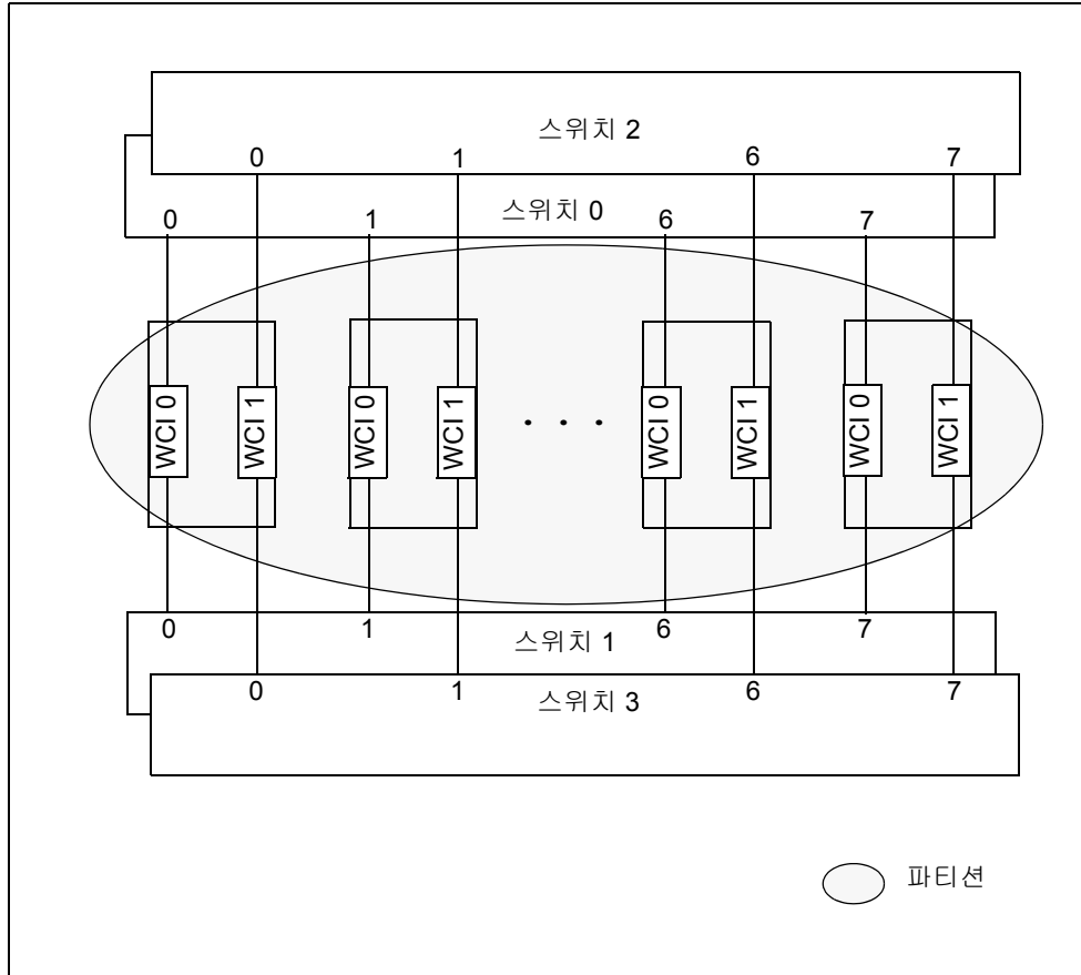
그림 6-2 단일 컨트롤러 예 - 여덟 개의 노드, 네 개의 스위치, 노드당 하나의 RSM 컨트롤러
