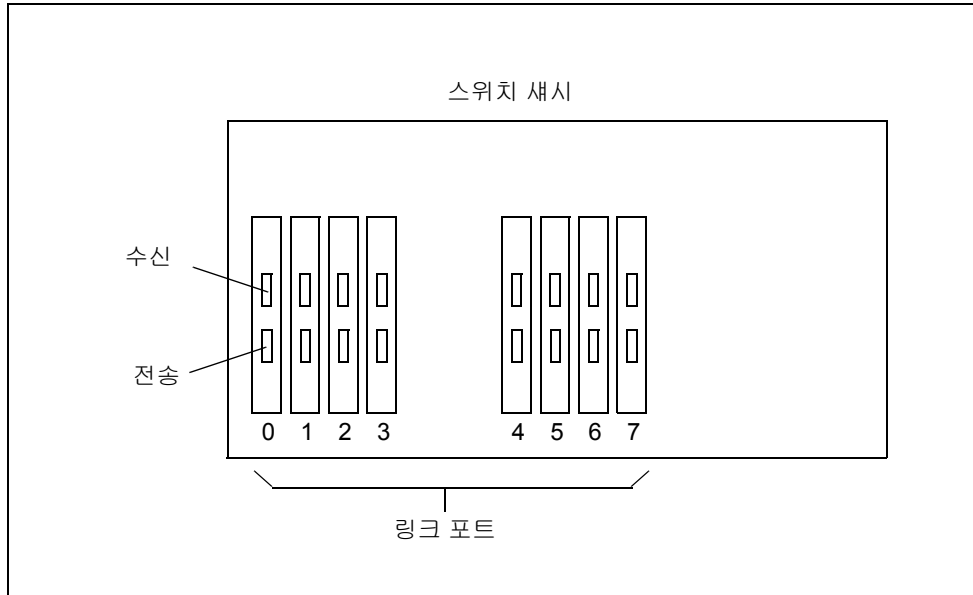
그림 10-4 Sun Fire Link 스위치의 광 포트 위치
