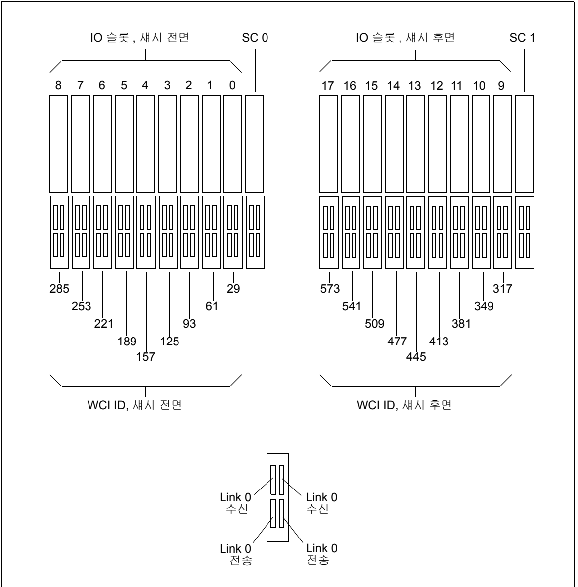
그림 10-3 Sun Fire 15K/12K 새시에 있는 Sun Fire Link 광 포트 위치
