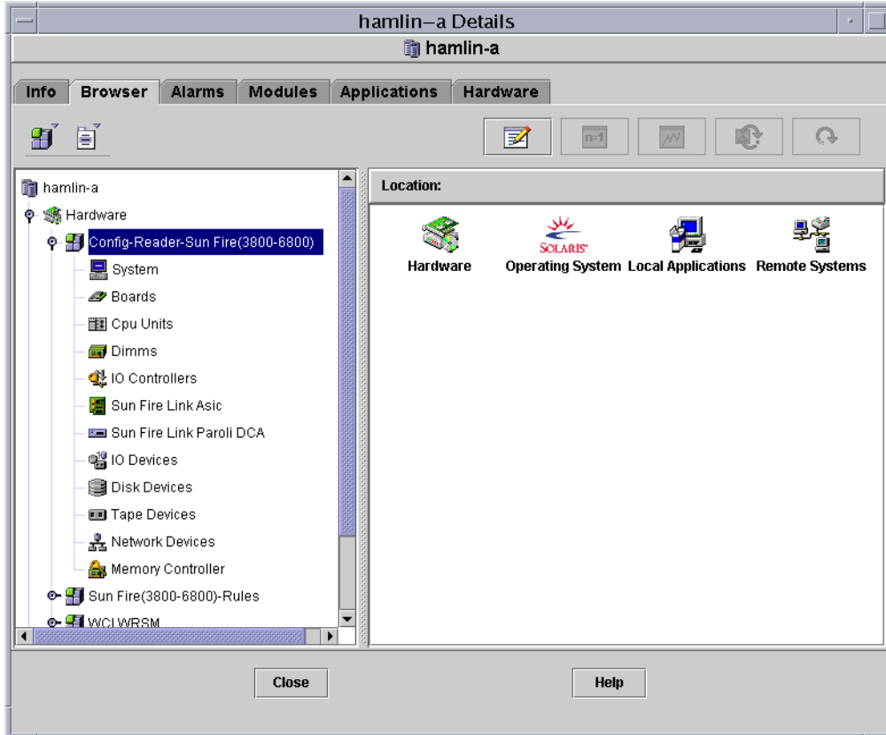
그림 9-9 Config-Reader 트리
