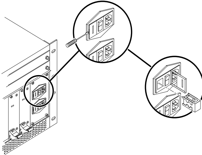
FIGURE 4-8 Remplacement d'un fusible dans l'unité d'entrée CA
