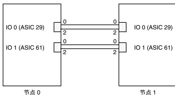
图 2-15 采用四路分割的两节点直接连接
