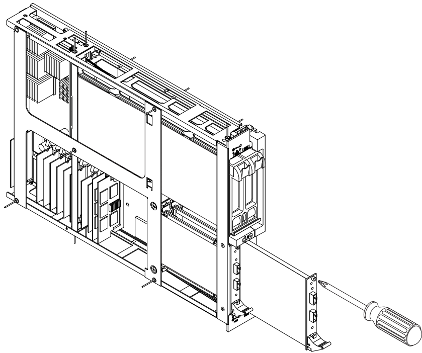
图 4-6 在 Sun Fire Link 配件中替换光学模块（Sun Fire 15K/12K 系统）
