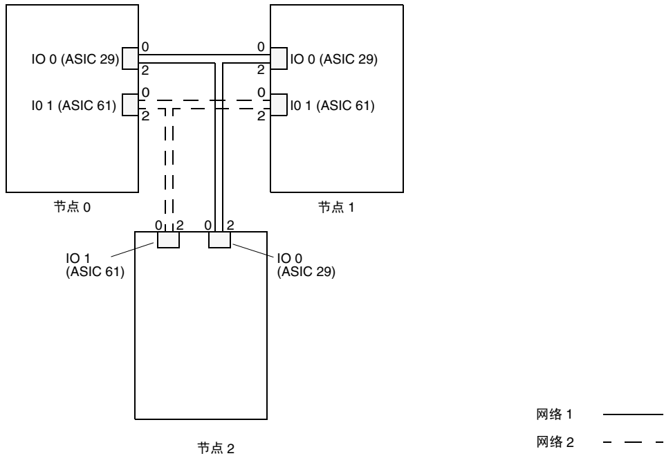
图 2-18 Sun 群集配置三节点直接连接中的两个网络
