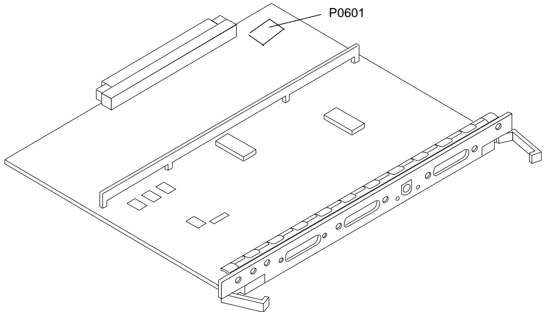
FIGURA 6-3 Posizione del jumper P0601 sulla scheda di clock
