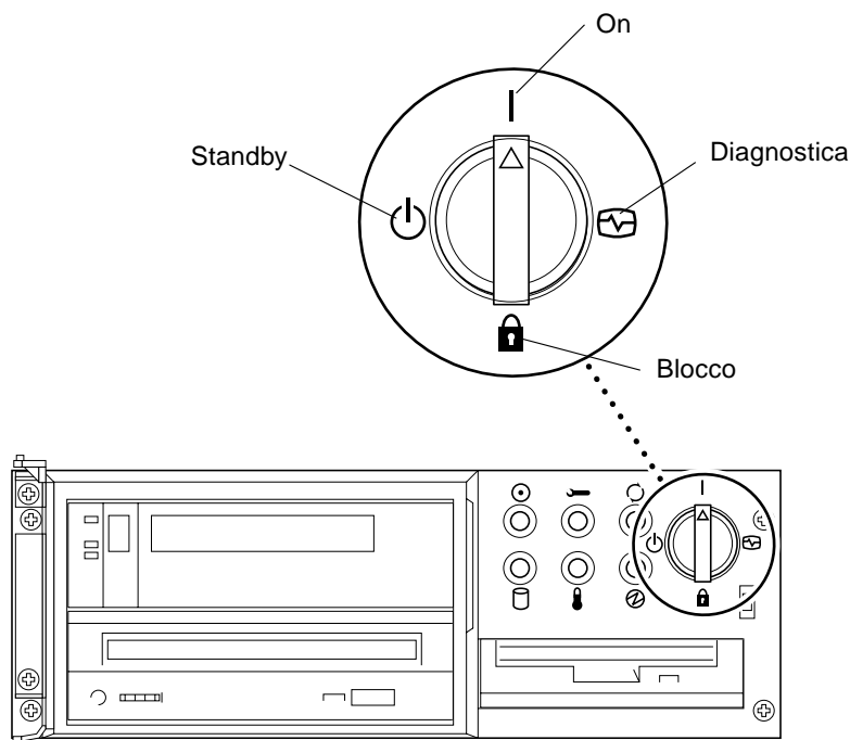
FIGURA 5-4 Posizioni degli interruttori a chiave sui sistemi Sun Enterprise 450 e Sun Ultra 450
