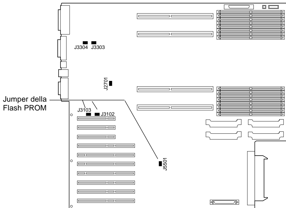
FIGURA 5-7 Posizione dei jumper della Flash PROM sui sistemi Sun Enterprise 450 e sulle workstation Sun Ultra 450
