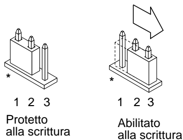
FIGURA 5-8 Impostazione del jumper J3103 di protezione/abilitazione alla scrittura sui sistemi Sun Enterprise 450 o Ultra 450
