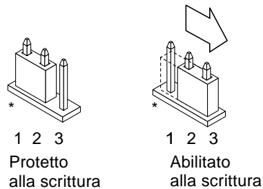
FIGURA 5-3 Impostazione del jumper di protezione/abilitazione alla scrittura nella posizione di abilitazione alla scrittura
