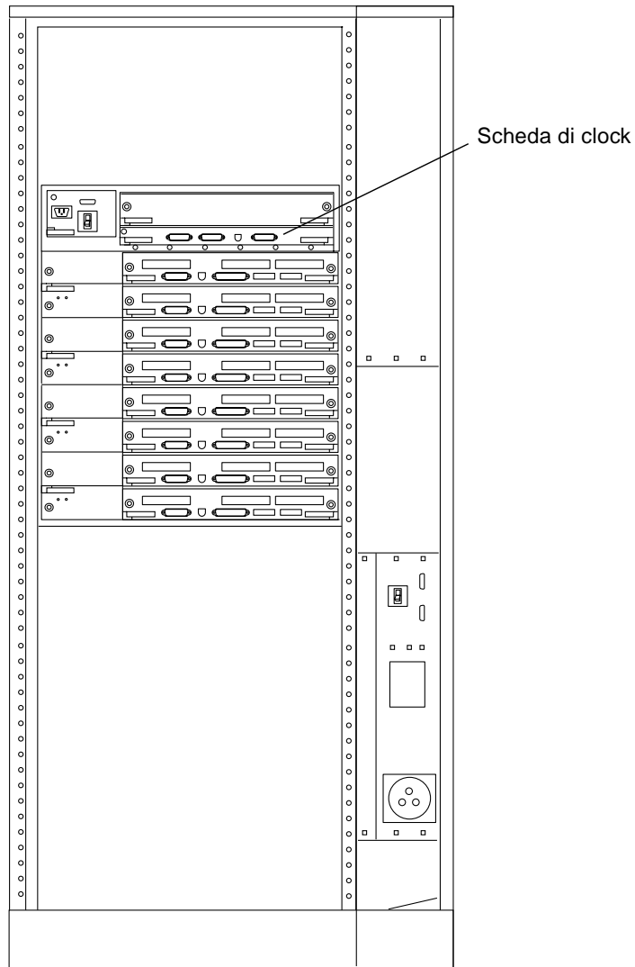
FIGURA 6-2 Vista posteriore del sistema Sun Enterprise 6000
