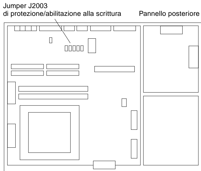
FIGURA 5-2 Posizione del jumper di protezione/abilitazione alla scrittura sulla scheda madre dei sistemi Sun Ultra 2
