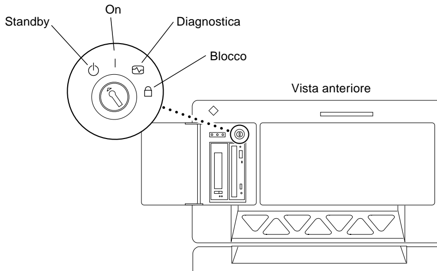
FIGURA 6-1 Posizione degli interruttori a chiave sui sistemi Sun Enterprise 6x00, 5x00, 4x00, 3x00
