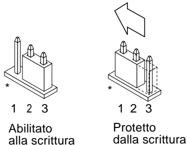
FIGURA 5-5 Impostazione del jumper di protezione/abilitazione alla scrittura in posizione protetta
