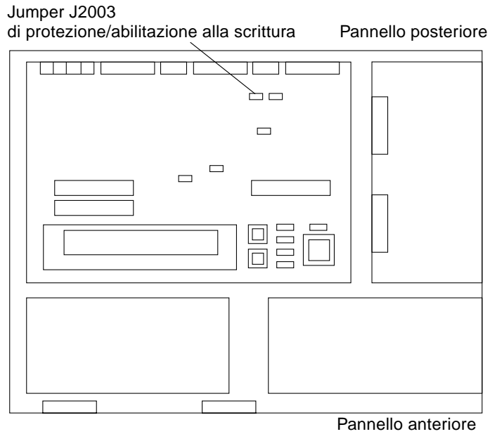
FIGURA 5-1 Posizione del jumper di protezione/abilitazione alla scrittura sulla scheda madre dei sistemi Sun Ultra 1
