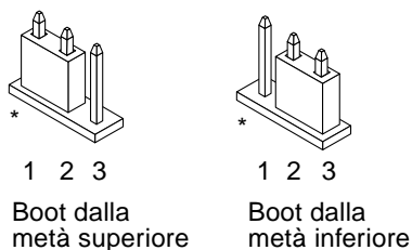
FIGURA 5-6 Impostazione del jumper di controllo del boot per l'esecuzione del boot dalla metà inferiore o dalla metà superiore
