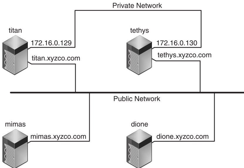
圖 5-2 網路介面
