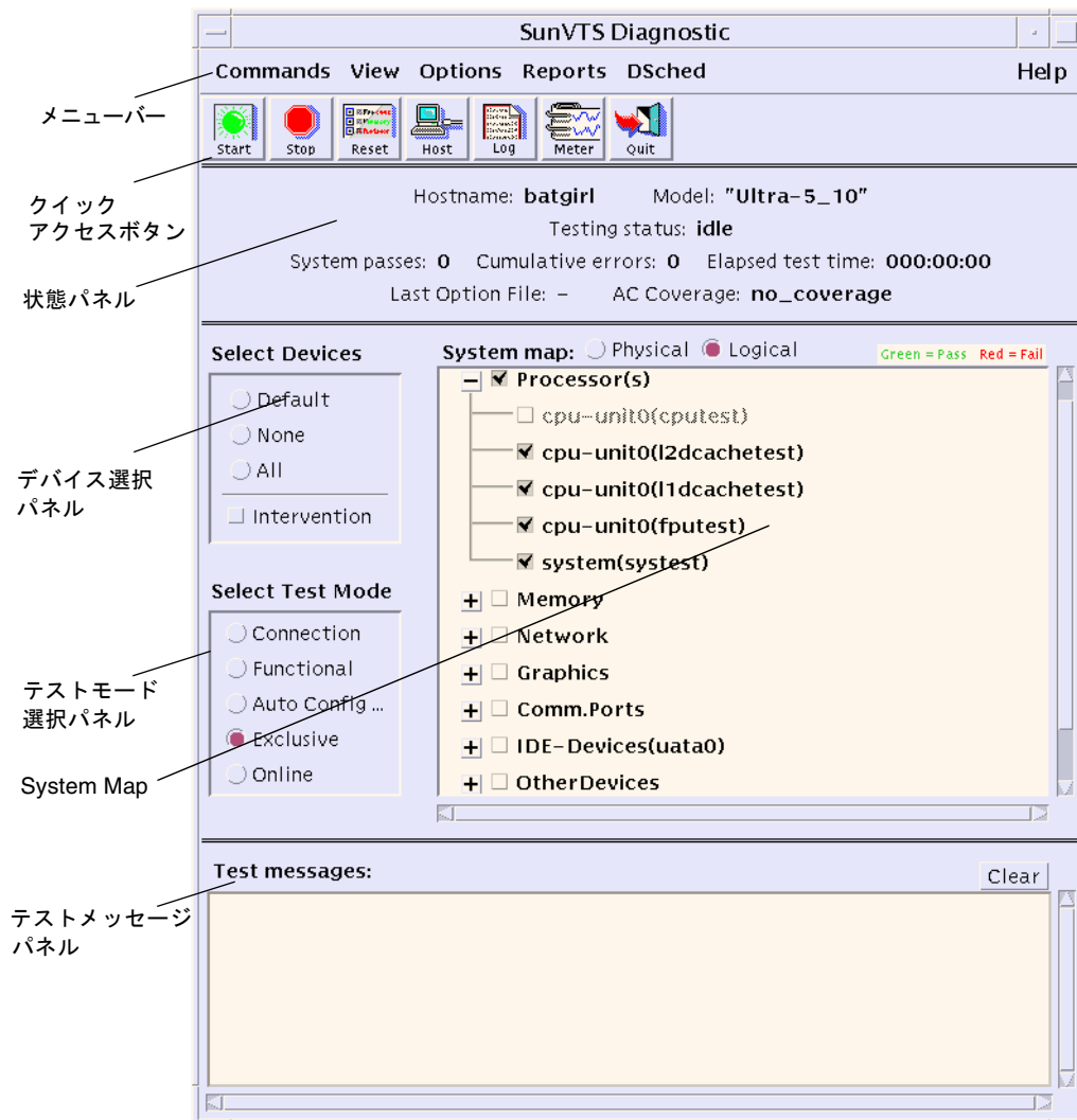
図 1-1 SunVTS CDE メインウィンドウ
