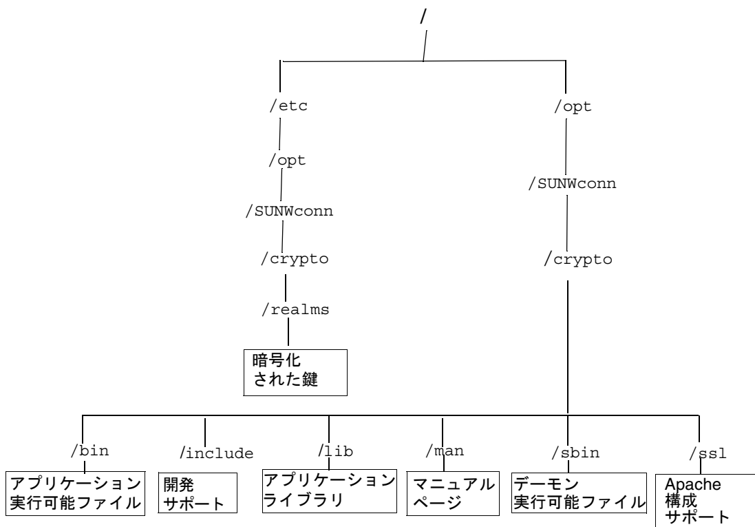
図 2-1 Sun Crypto Accelerator 1000 のディレクトリおよびファイル
