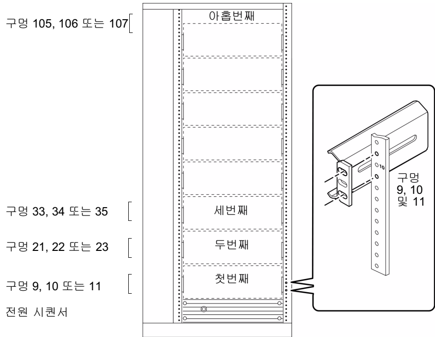
36 RU 캐비닛에 있는 9 개 서버의 앞면 모양
