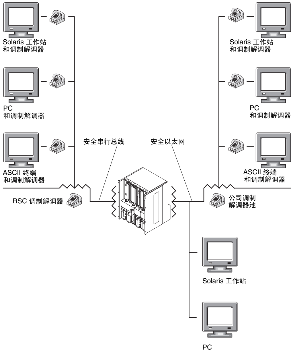
图 1-1 RSC 远程访问路径
