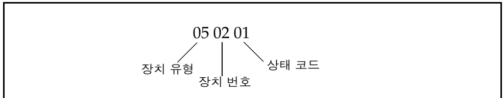
그림 3-1 메시지 형식
