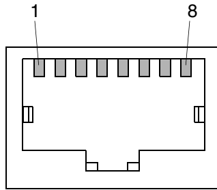
圖 5-27 RJ-45 乙太網路接頭圖
