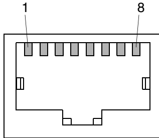
圖 5-24 RJ-45 乙太網路接頭圖
