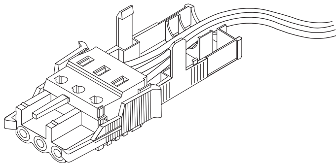
圖 5-52 從應力消除盒底部拉出電線
