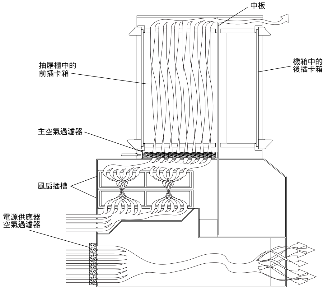
圖 2-14 氣流（側面圖）
