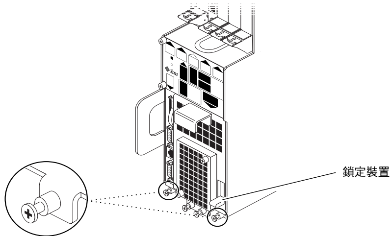
圖 2-11 鬆開 Netra ct 400 伺服器底部的螺絲
