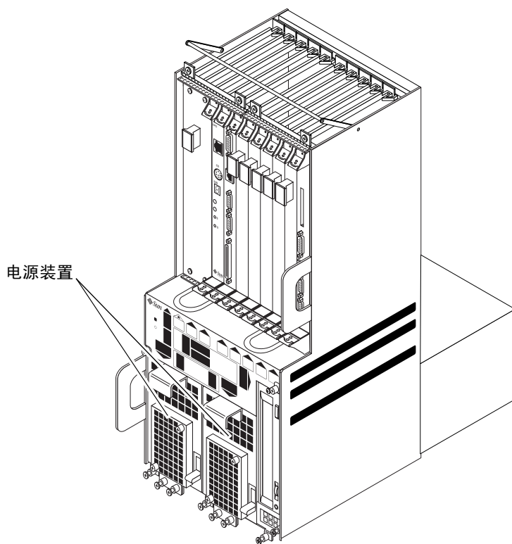
图 1-27 电源装置的位置 (Netra ct 800 服务器)
