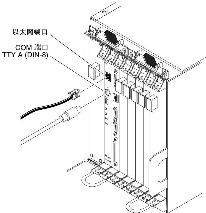
图 1-25 CPU 卡
