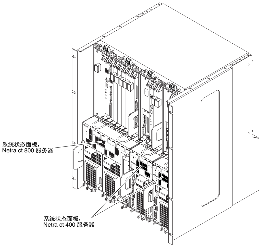
图 1-29 系统状态面板位置
