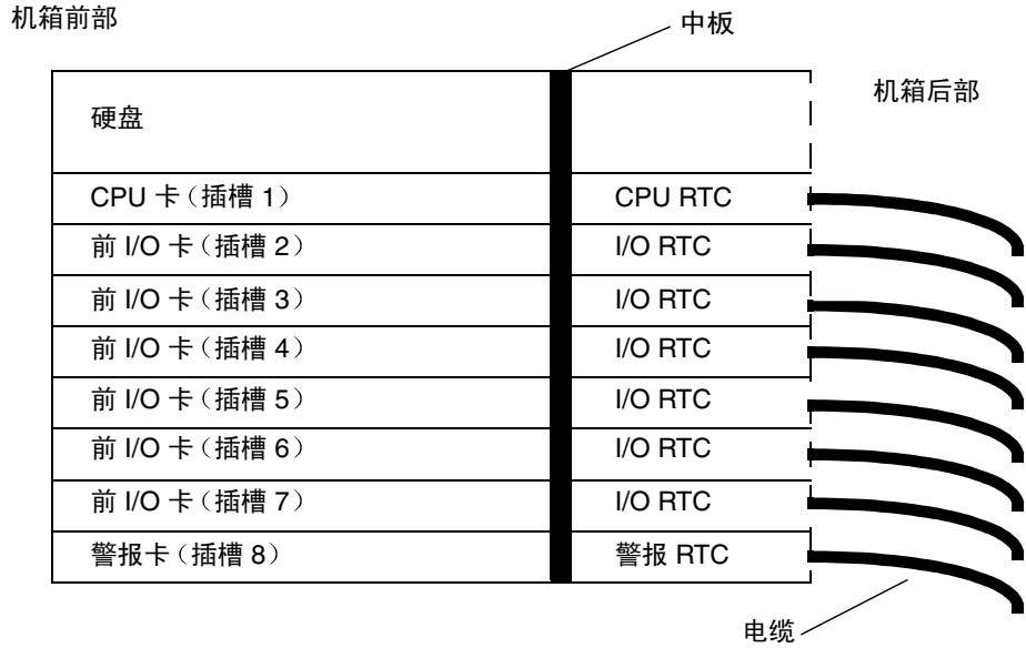
图 1-16 后连接型 Netra ct 800 服务器 (俯视图)
