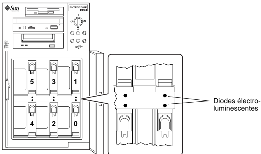
FIGURE 2-3 Numérotation des emplacements d'unité de disque et emplacement des diodes électroluminescentes
