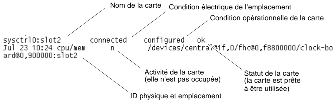
FIGURE 1-1 Détails de l'écran relatif à cfdm -v
