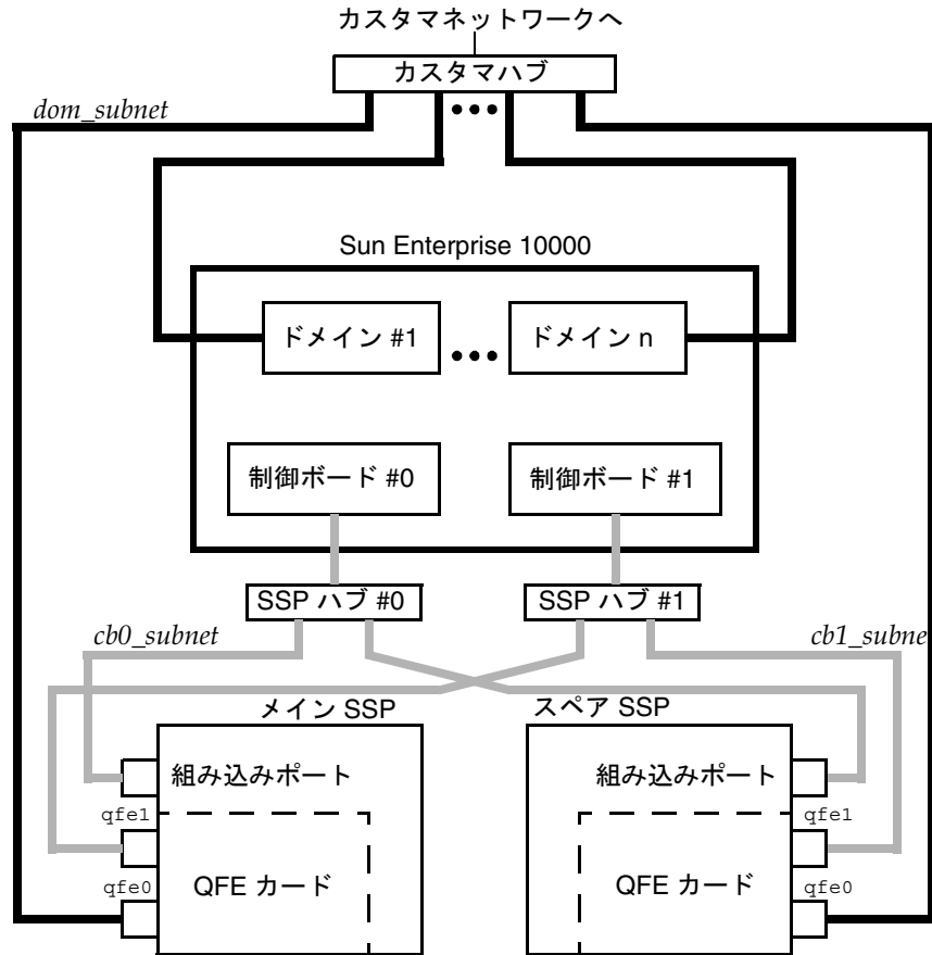
図 A-3 スペア SSP のネットワーク構成
